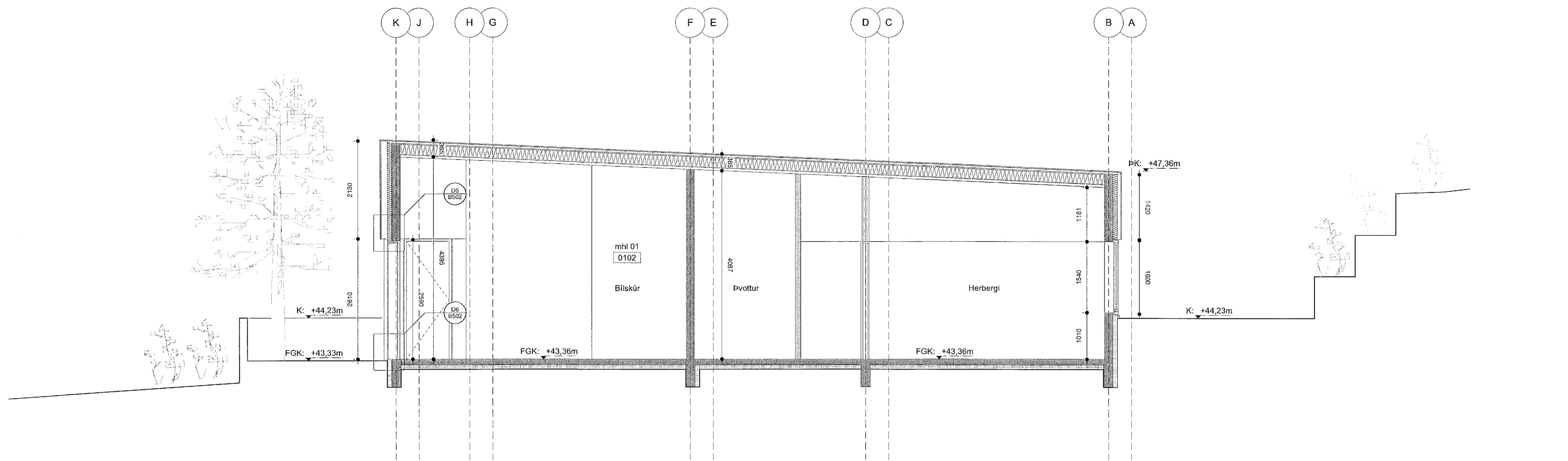
Sneiðing C-C mkv: 1:100
