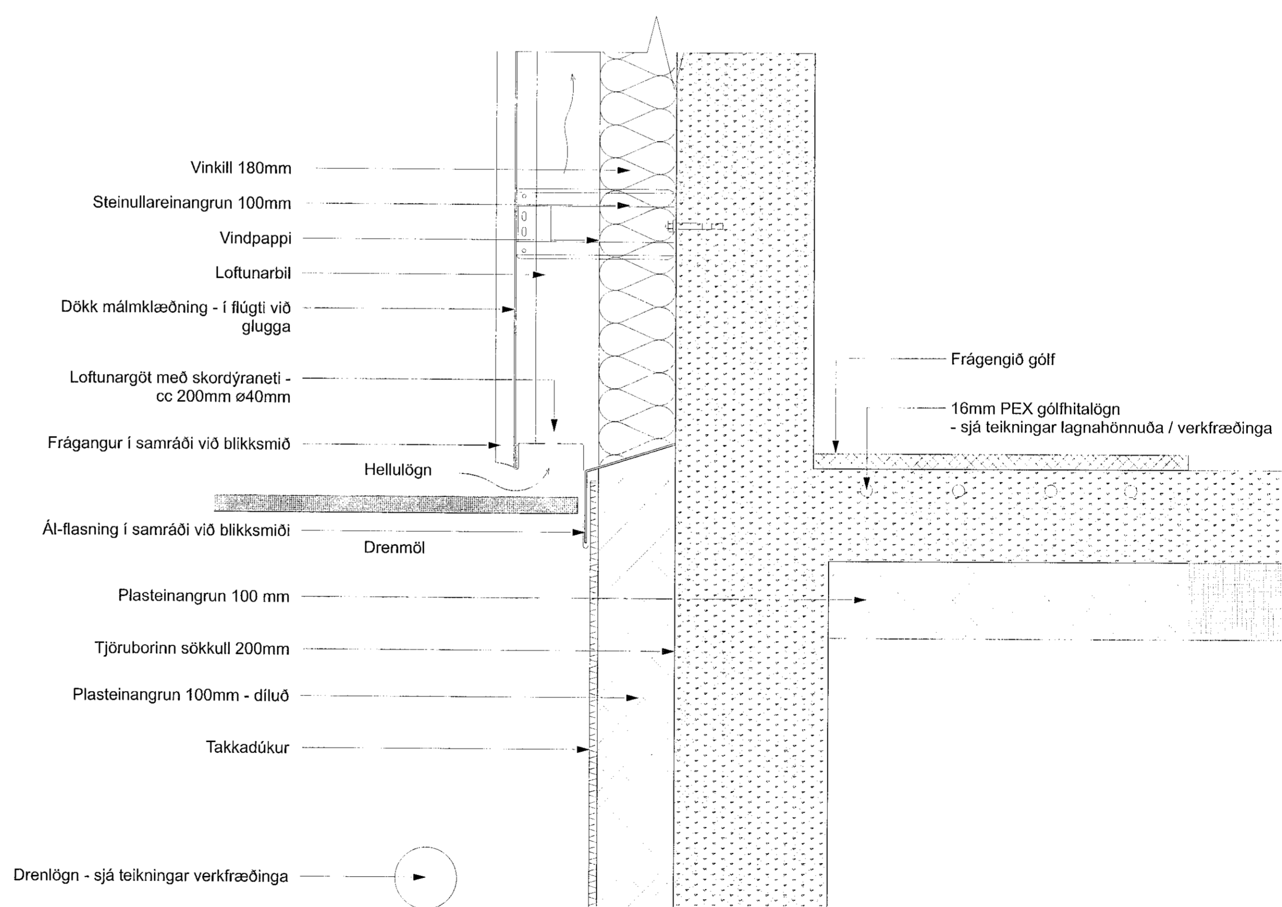
D-9 Deili í útvegg Sökkul / þakskyggni mkv. 1:5
