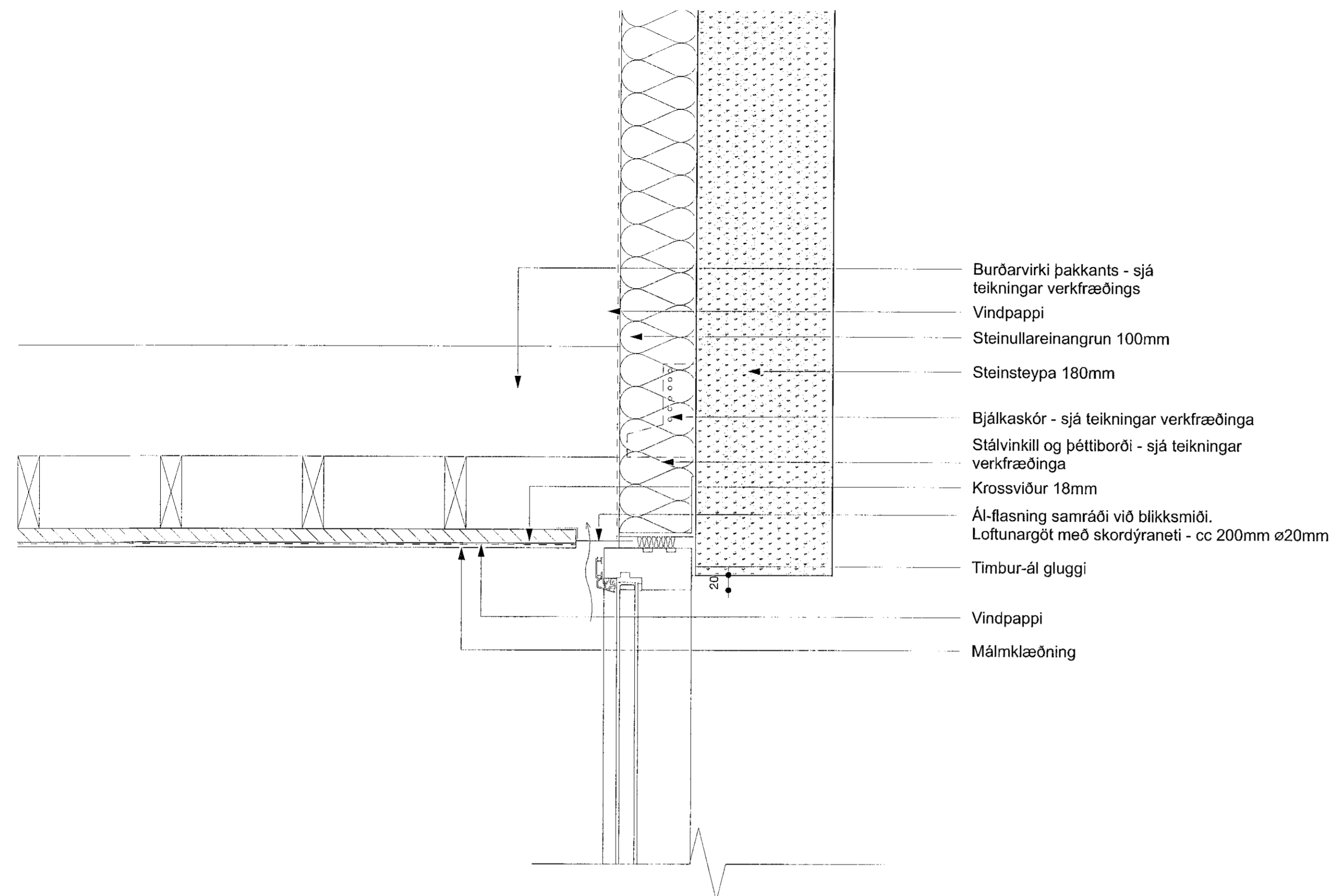
D-7 Deili í þakskyggni mkv. 1:5
