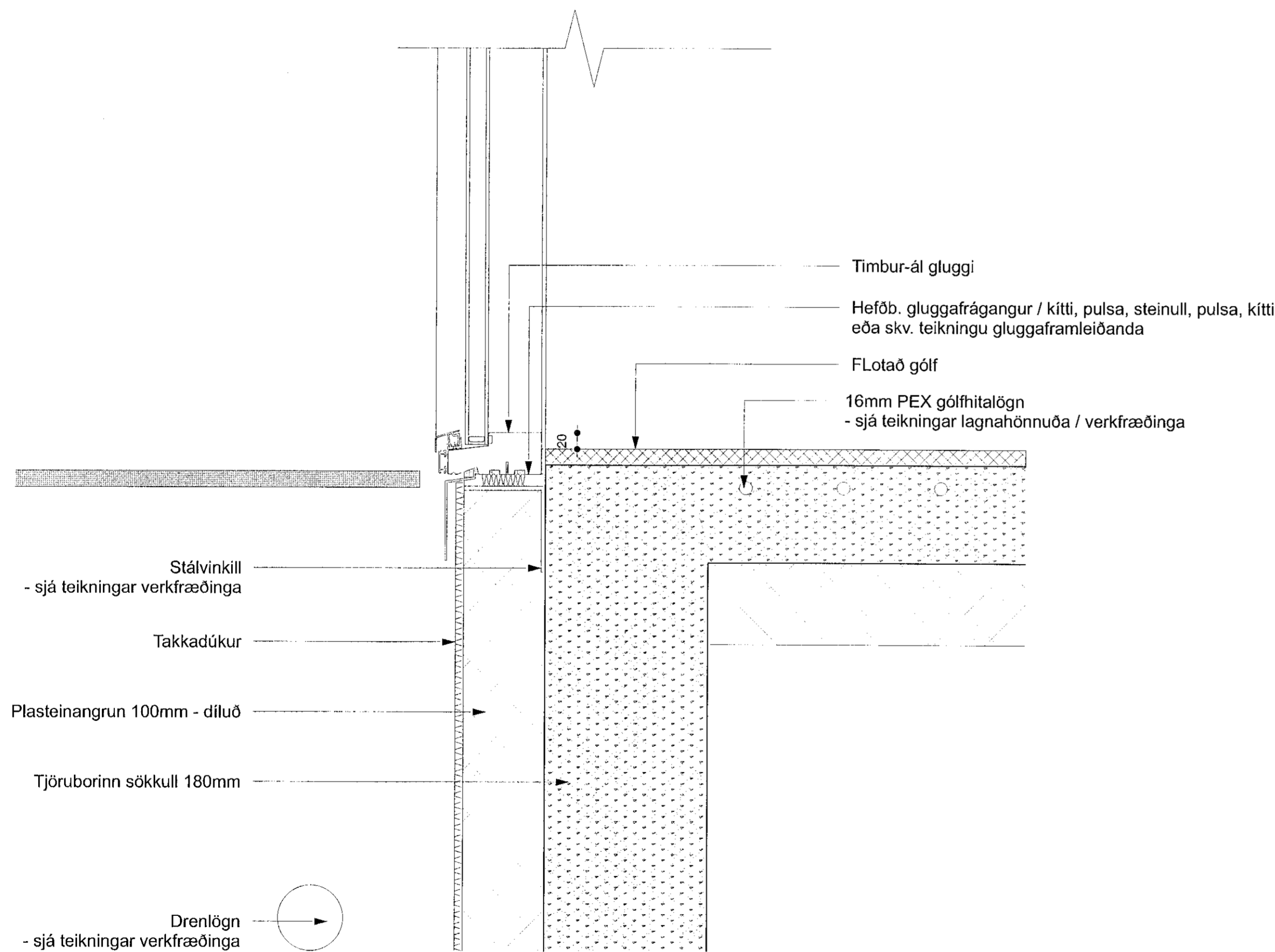
D-8 Deili í gólf, sökkul og glugga mkv. 1:5
