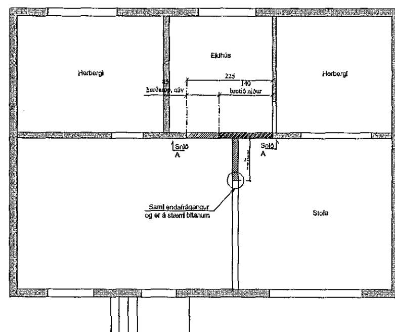
GRUNNMYND. 1:100
