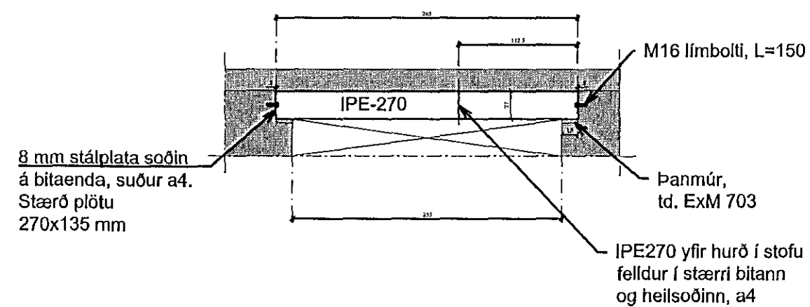
SNID A-A 1:50
