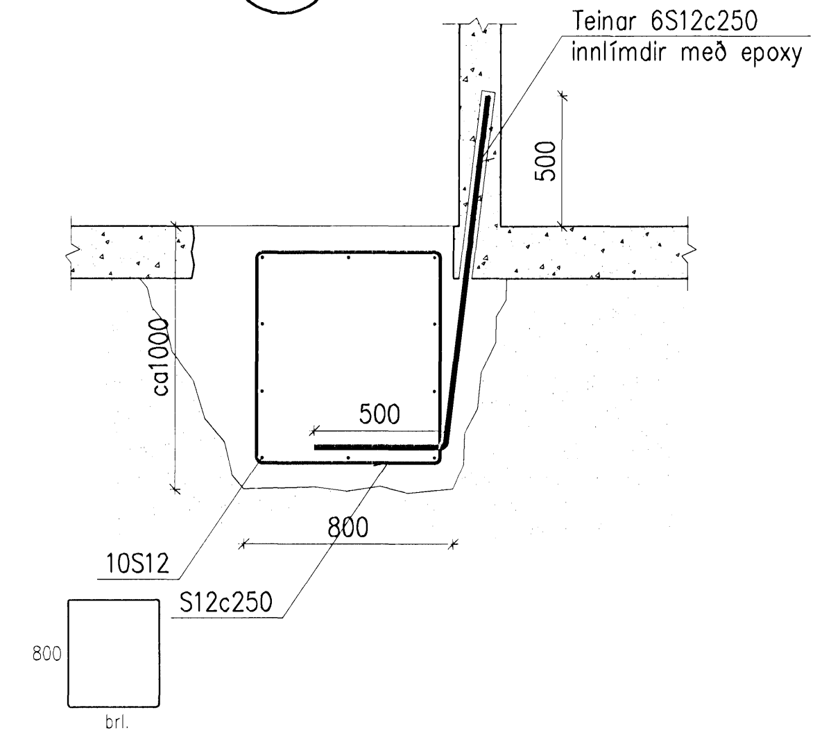
2 SNIÐ, 1:20
