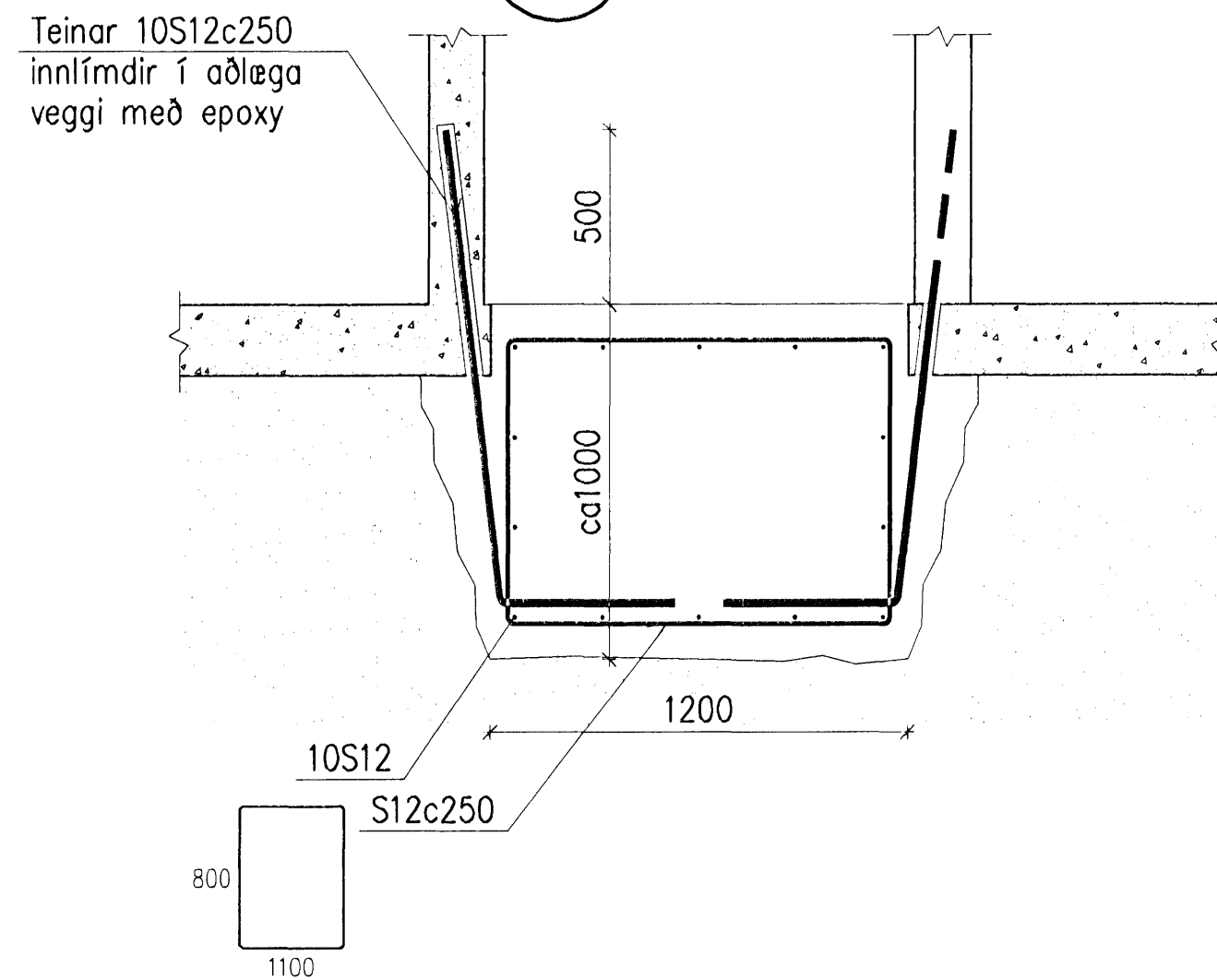
3 SNIÐ, 1:20
