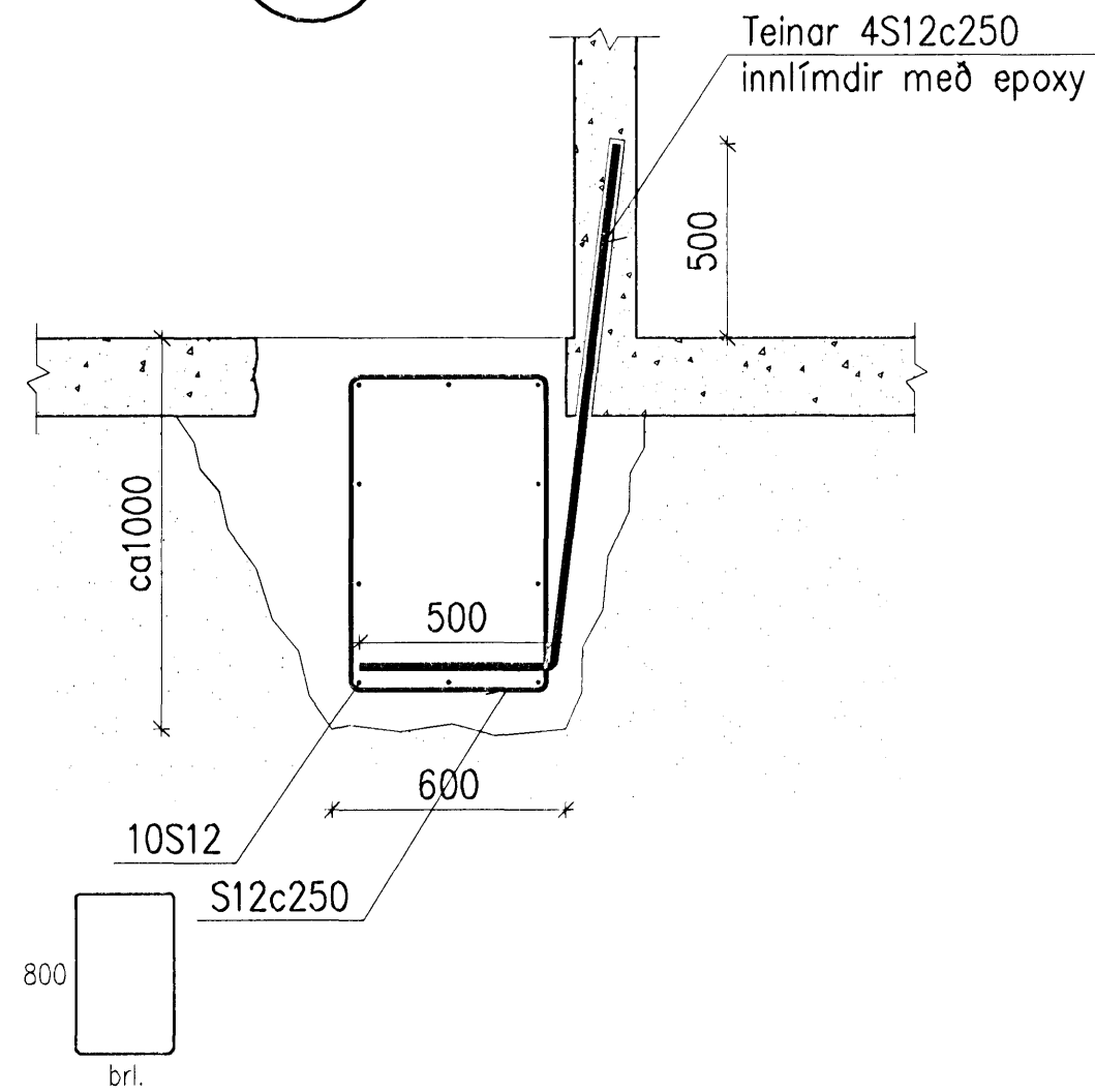
1 SNIÐ, 1:20
