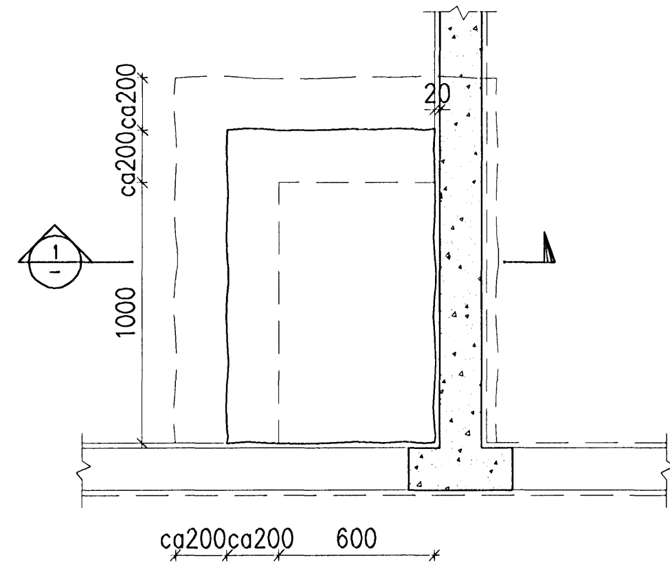
D1 DEILI, 1:20 394
