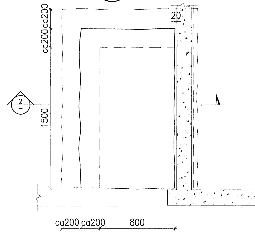
D2 DEILI, 1:20 394
