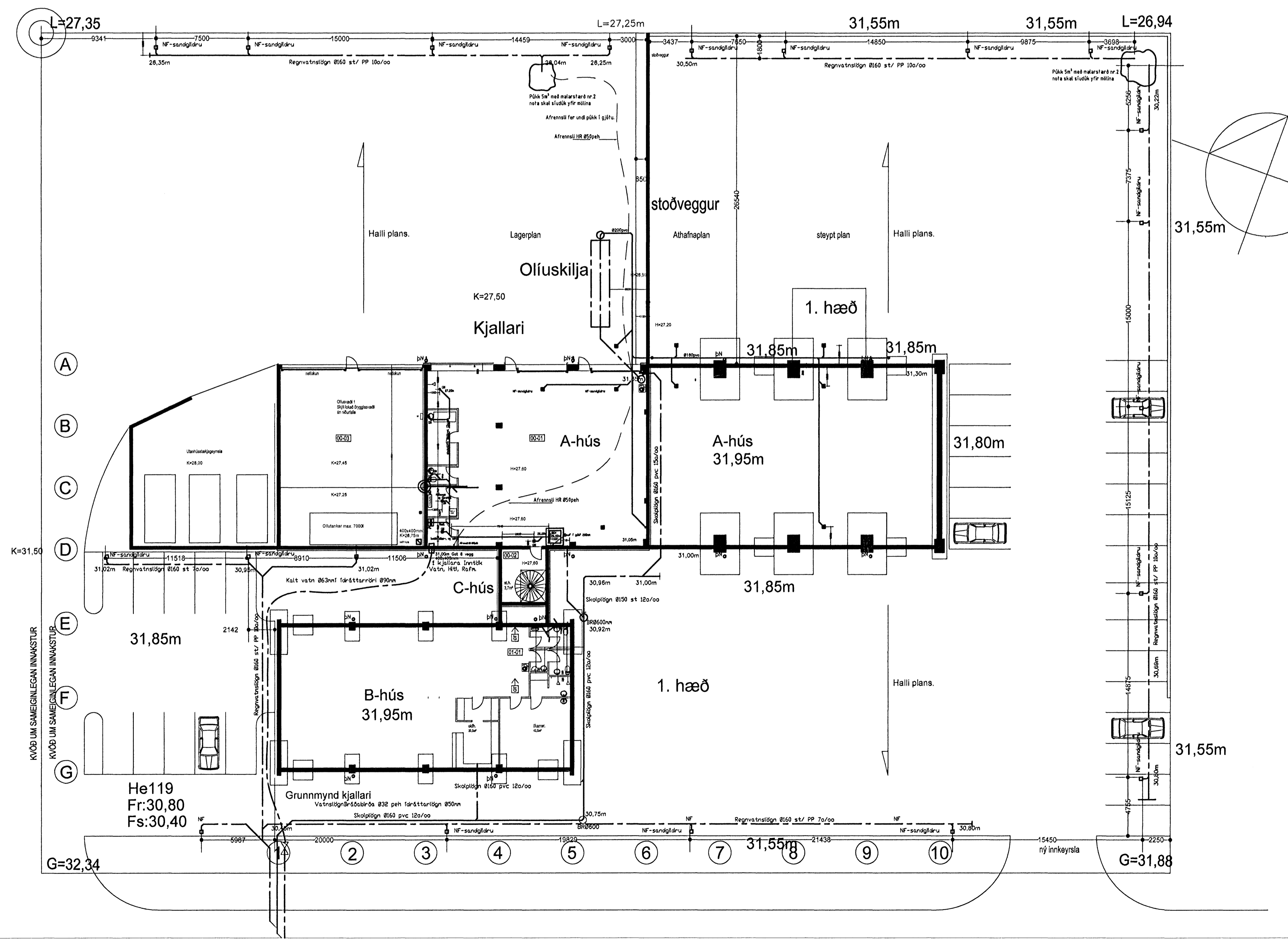
Yfirlitsmynd 1:200
