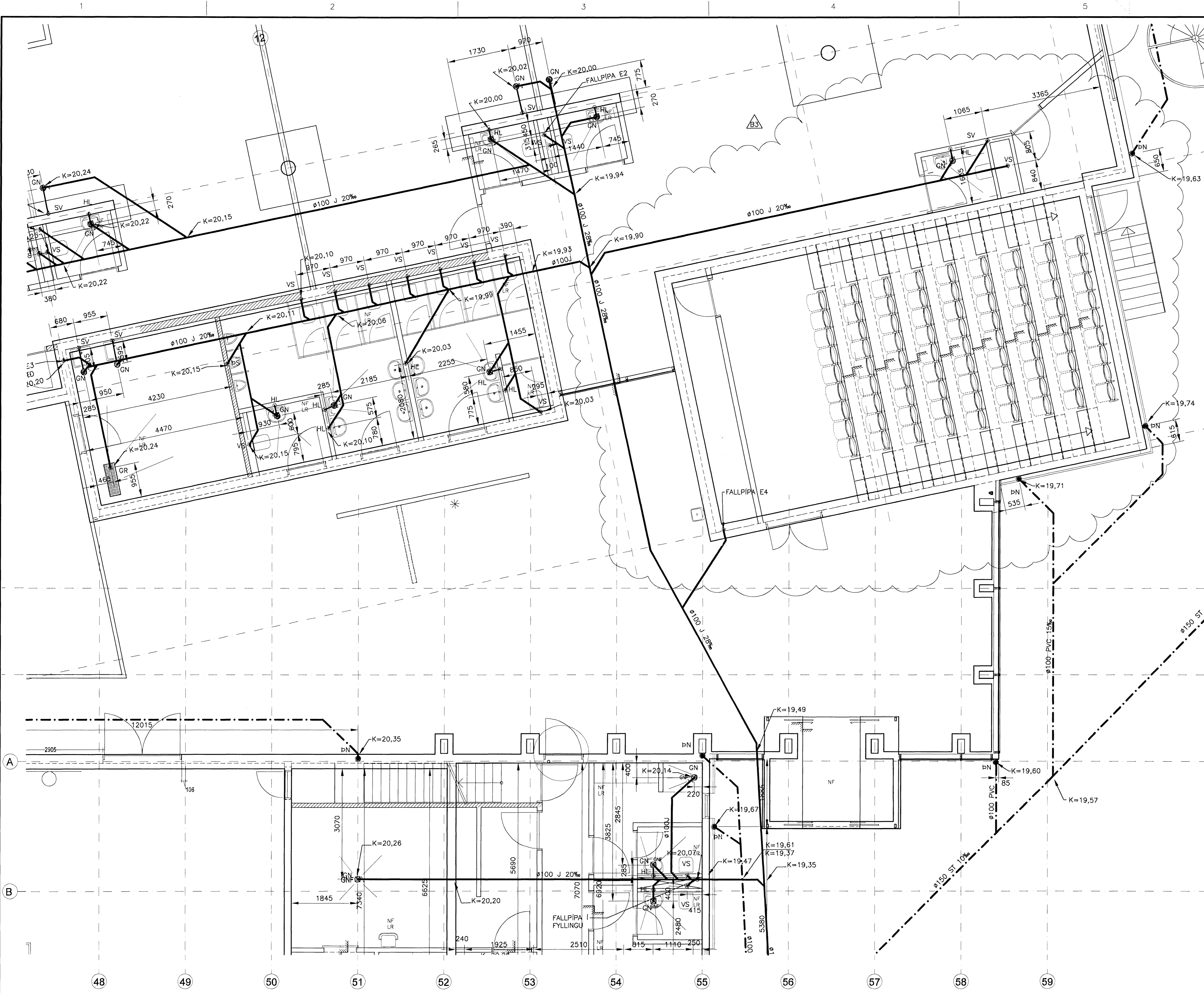
GRUNNMYND MKV. 1
