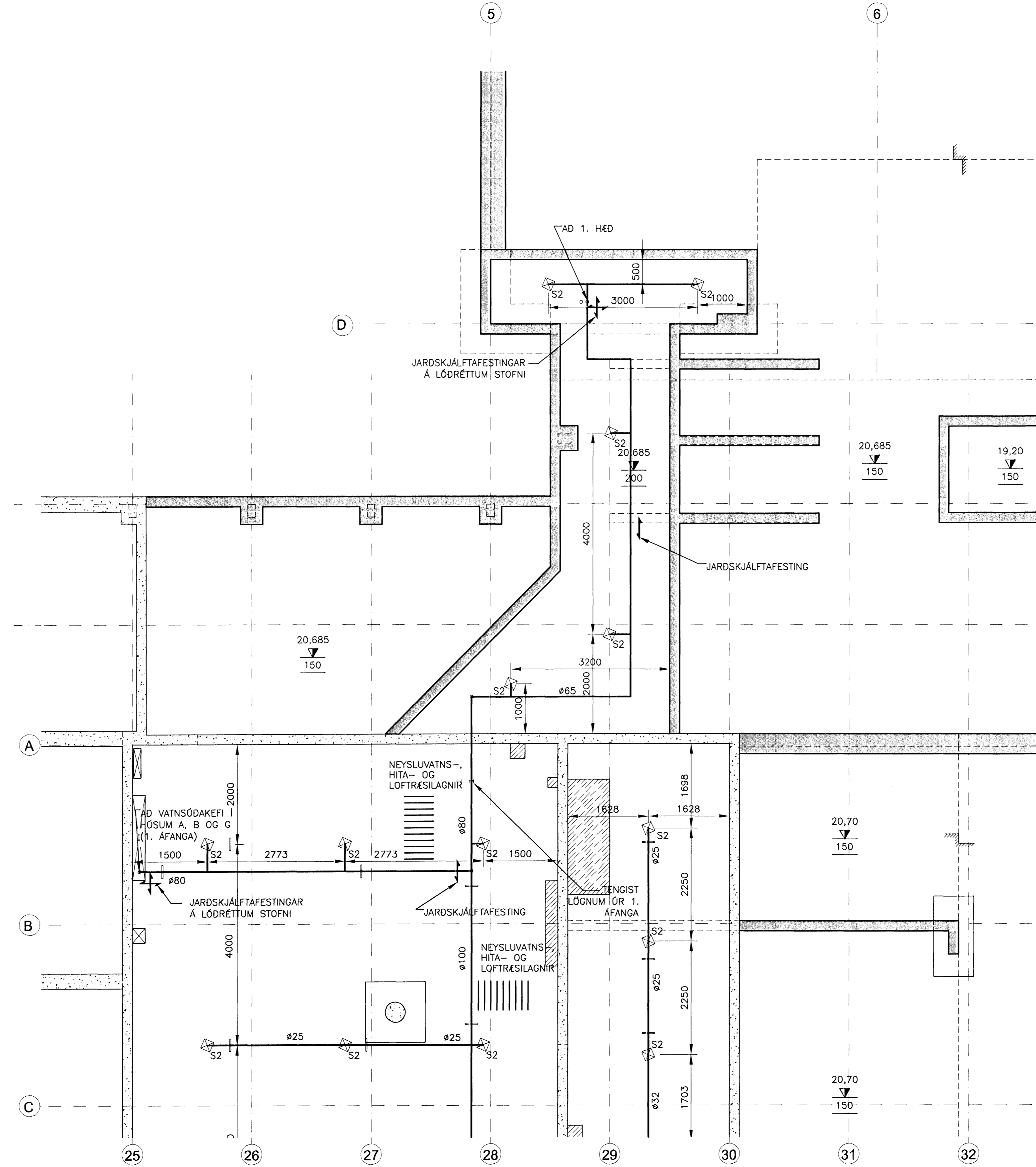
GRUNNMYND MKV. 1
