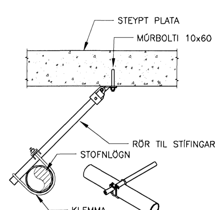
JARÐSKJÁLFTAFASTING, STÍFING Í 2 ÁTTIR (ÞVERT Á LEIDSLU). EKKI Í KVARDA
