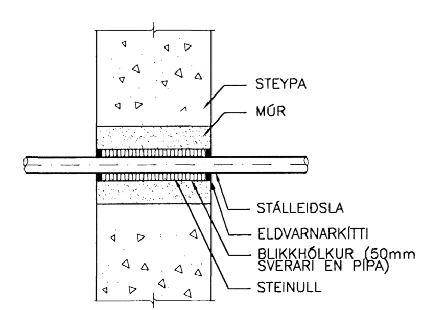
BRUNABÉTTING Á LEIDSLU GEGNUM STEYPTAN VEGG EKKI Í KVARDA
