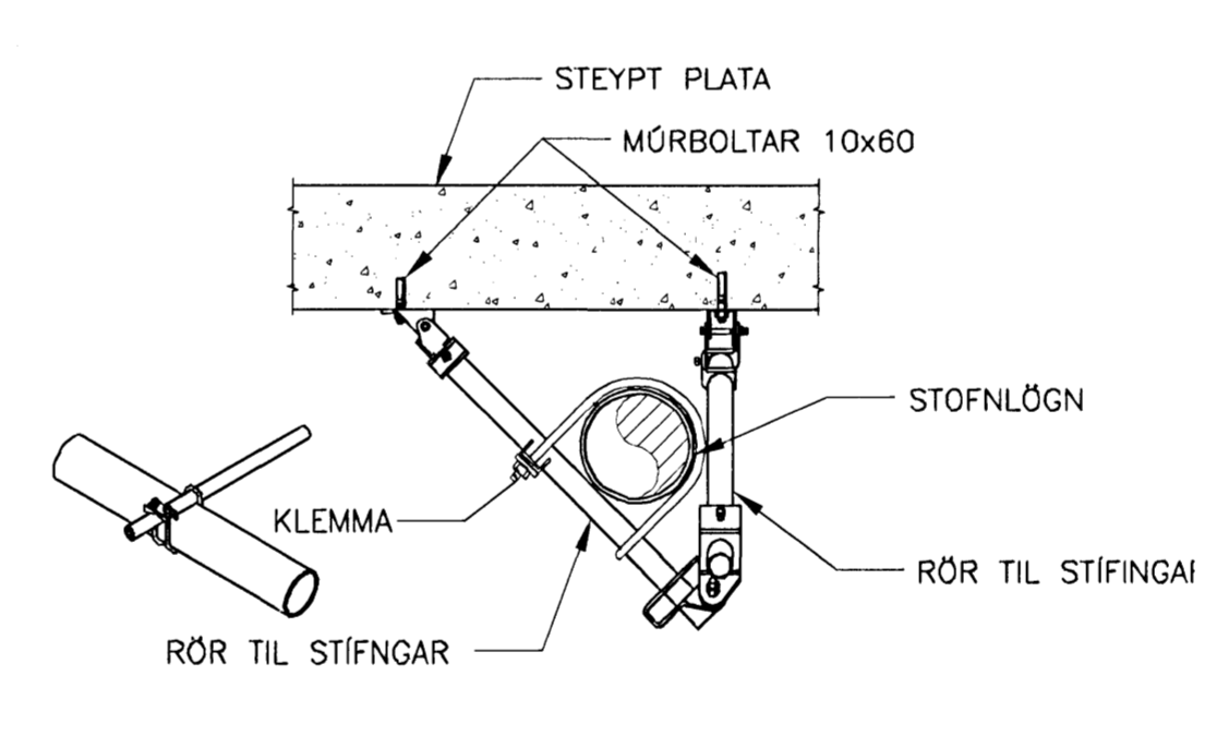
JARÐSKJÁLFTAFASTING, STÍFING Í 4 ÁTTIR EKKI Í KVARDA
