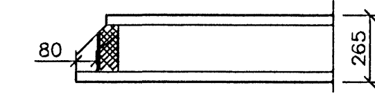
Snið í enda holplatna sem hvíla á steypum veggjum. Málkvarði 1:20
