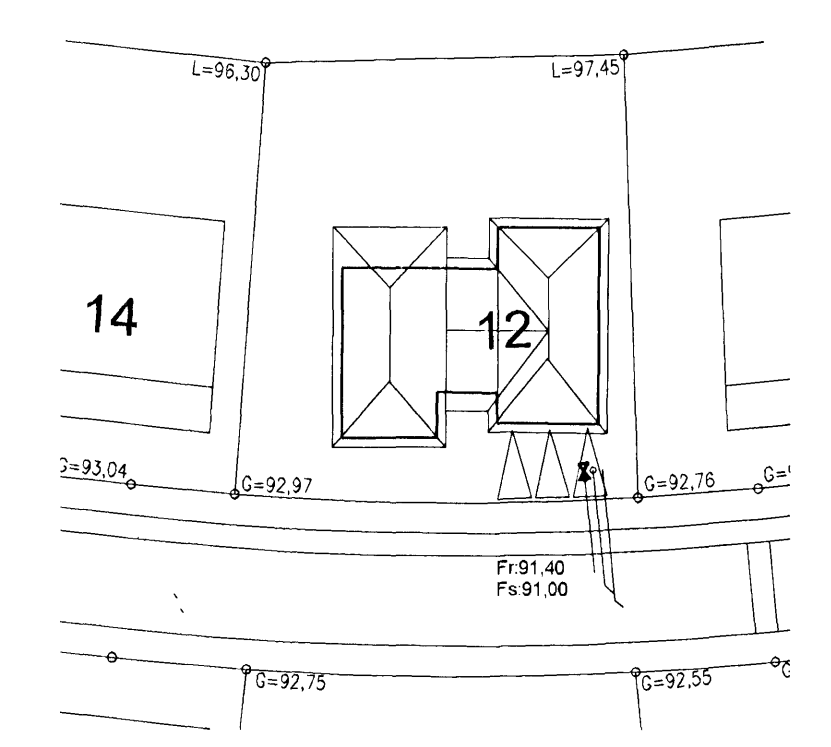
Afstöðumynd 1:500
