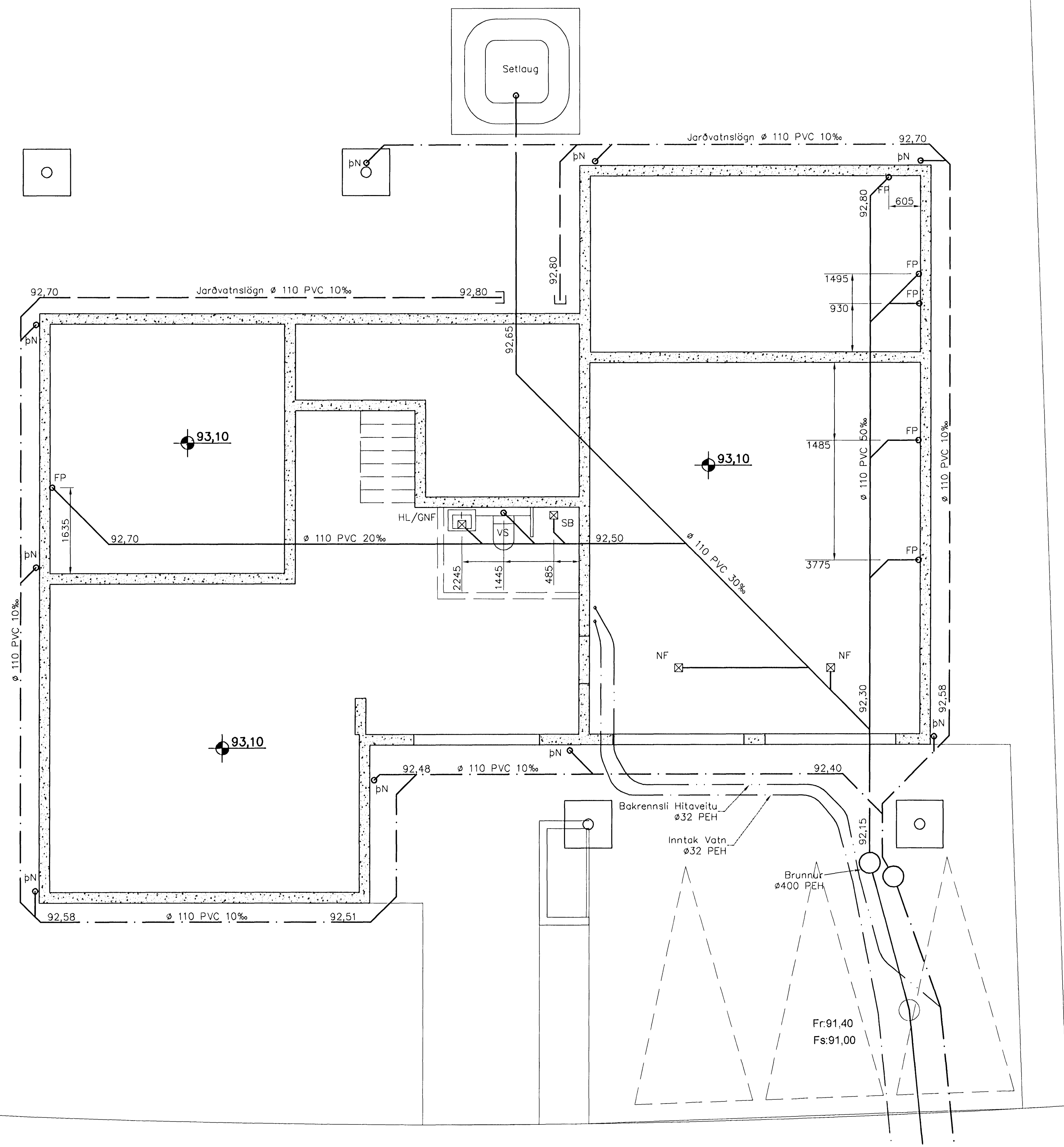
Grunnlagnir 1:50
