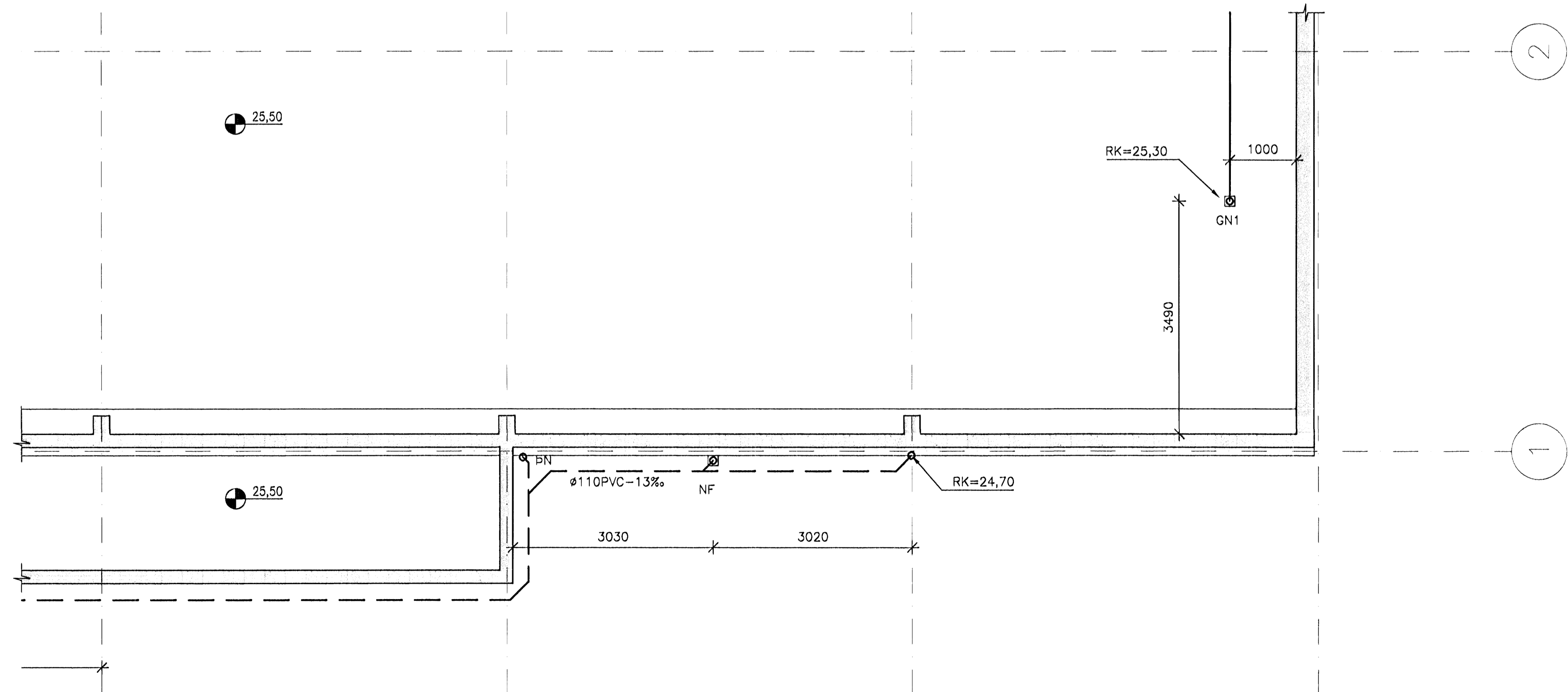
GR Grunnmynd 3 - 1:50
