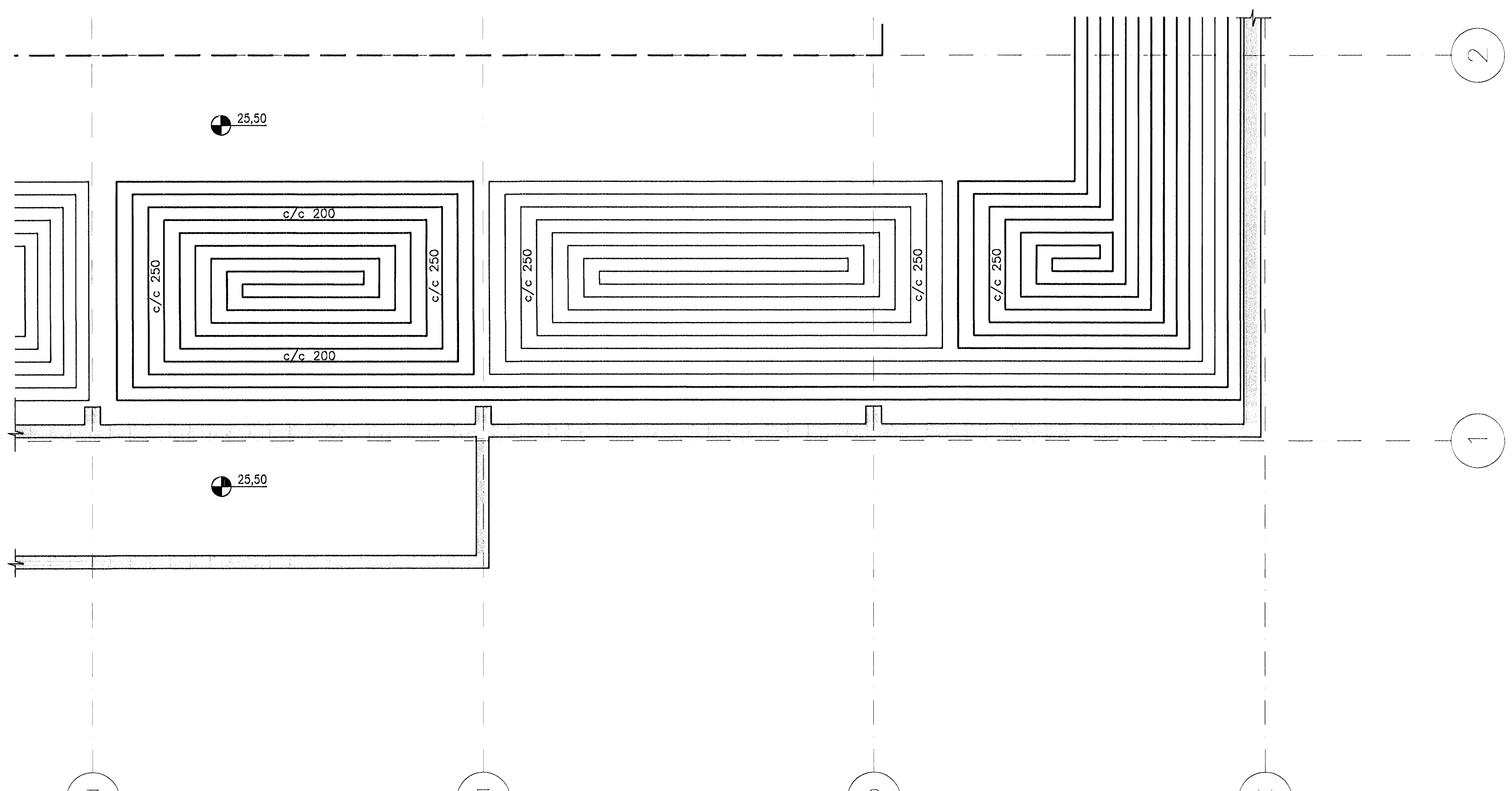
GR Grunnmynd 3 1:50
