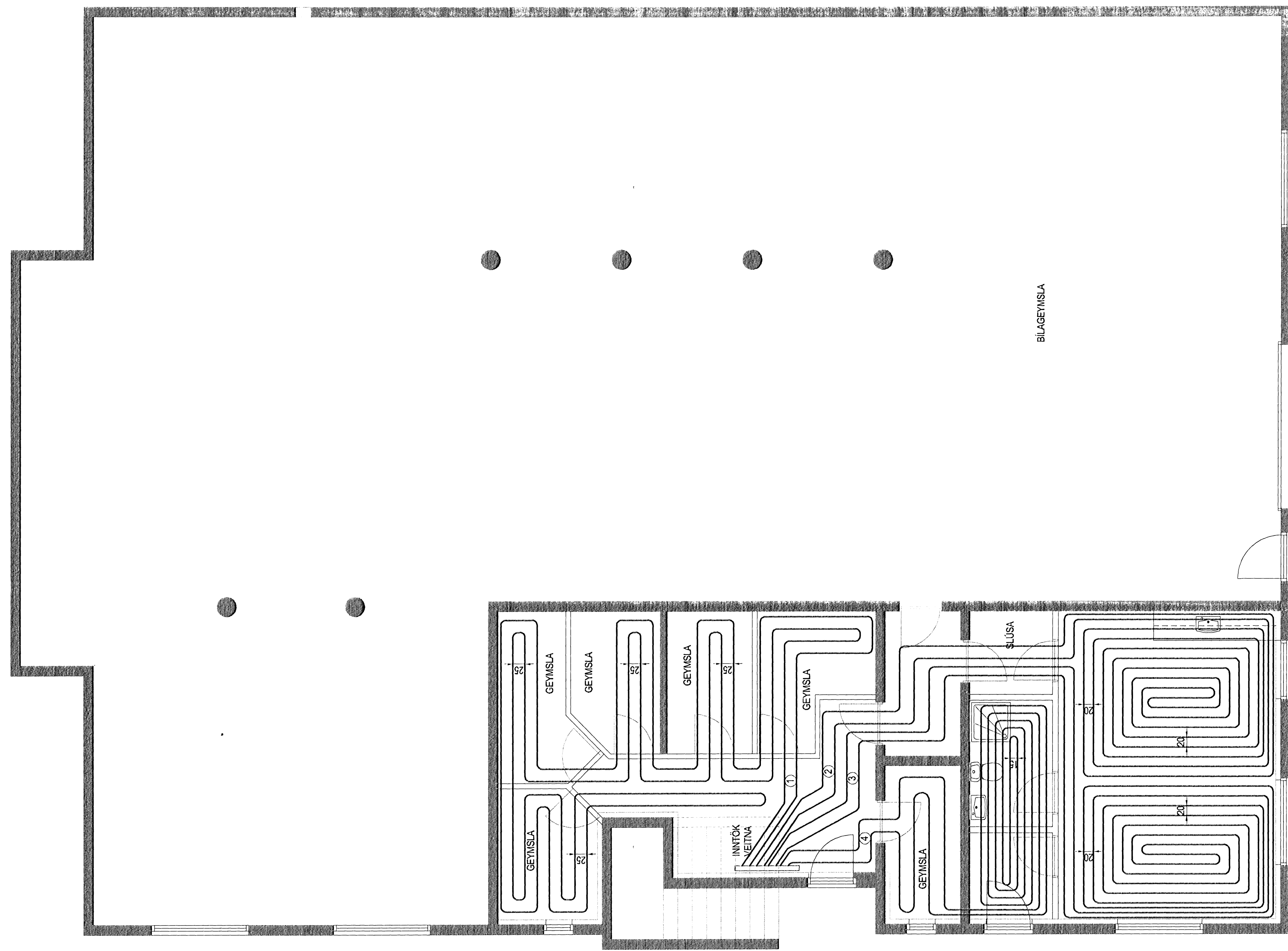
GÓLFHITALAGNIR, GRUNNMYND KJALLARA MKV. 1:50
