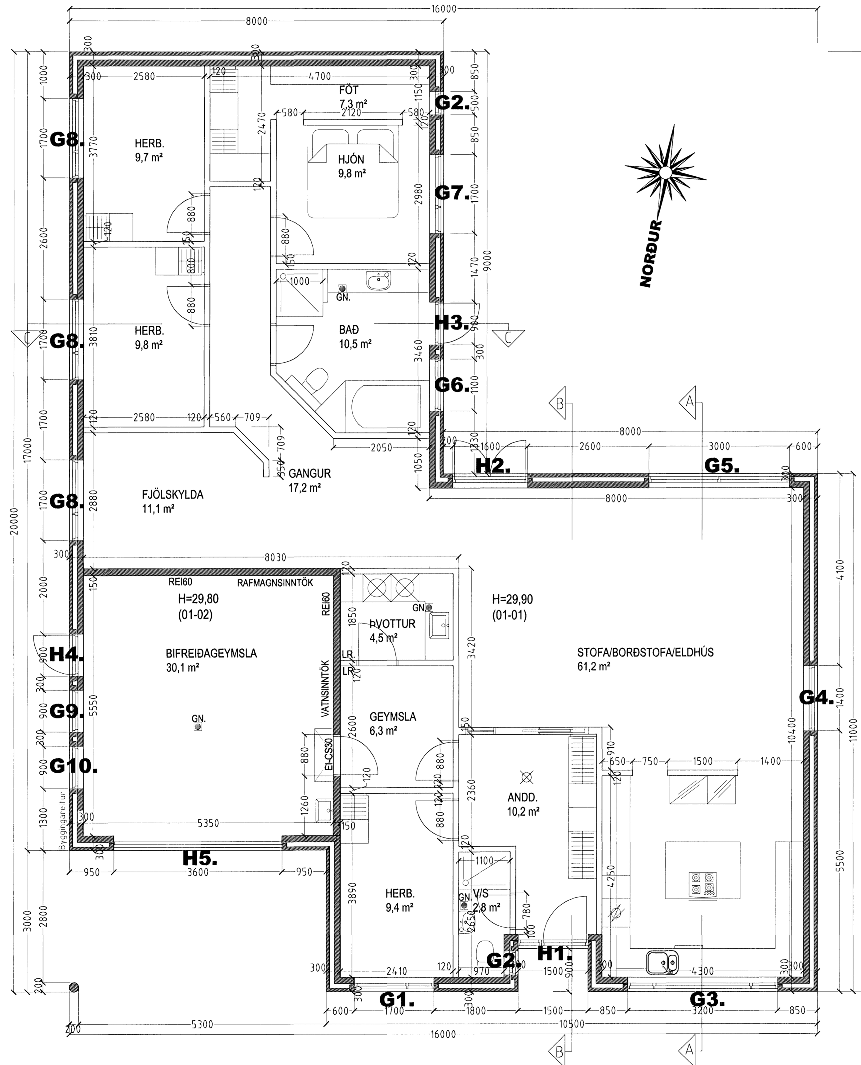
GRUNNMYND MKV. 1:50.
