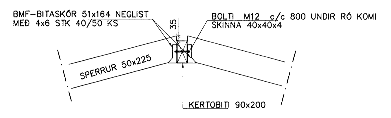
SNIÐ 2 1:20
