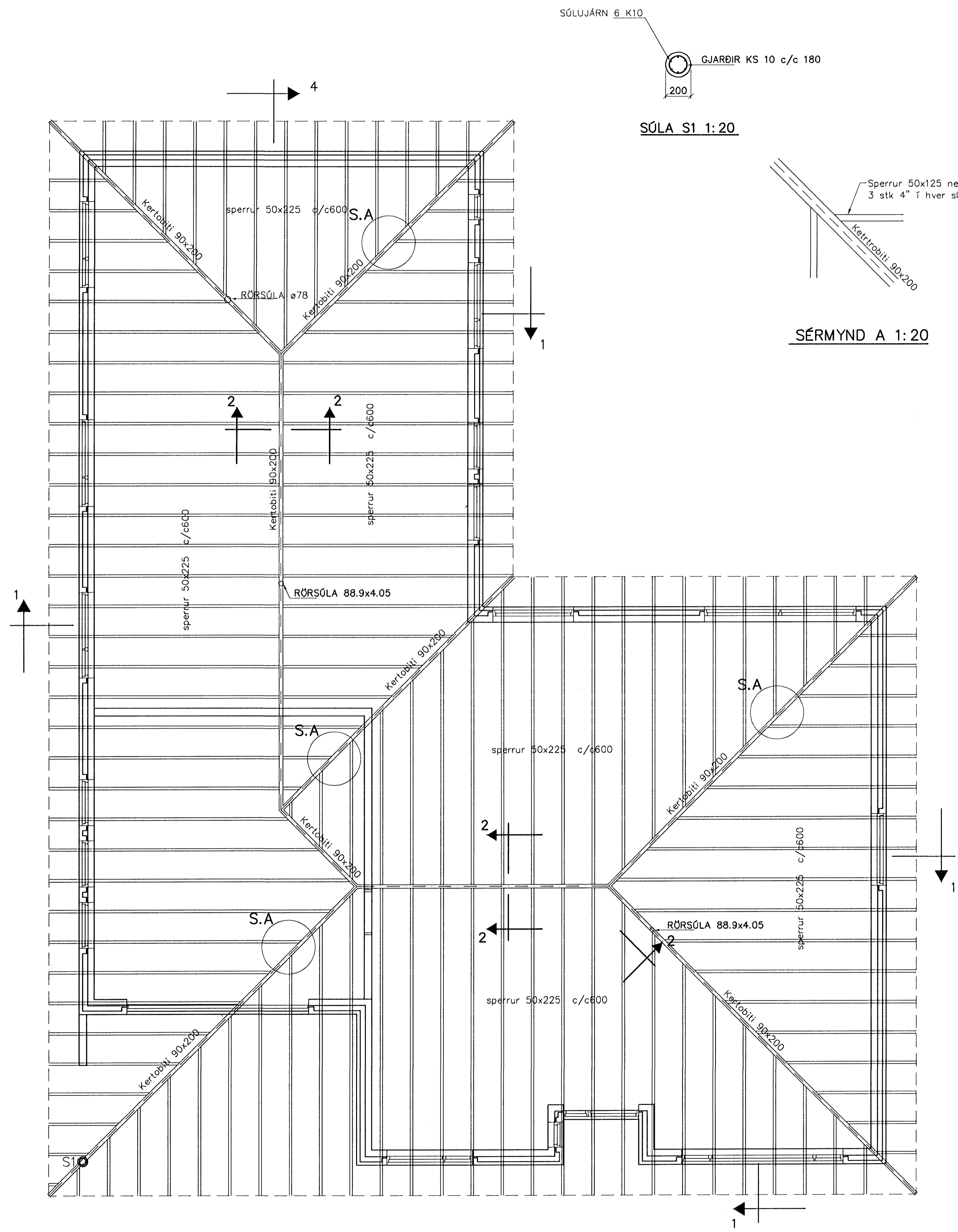
GRUNNMYND 1:50
