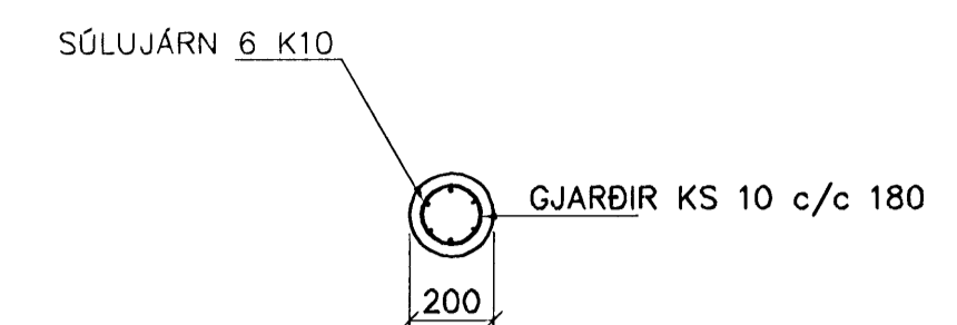
SÚLA S1 1:20
