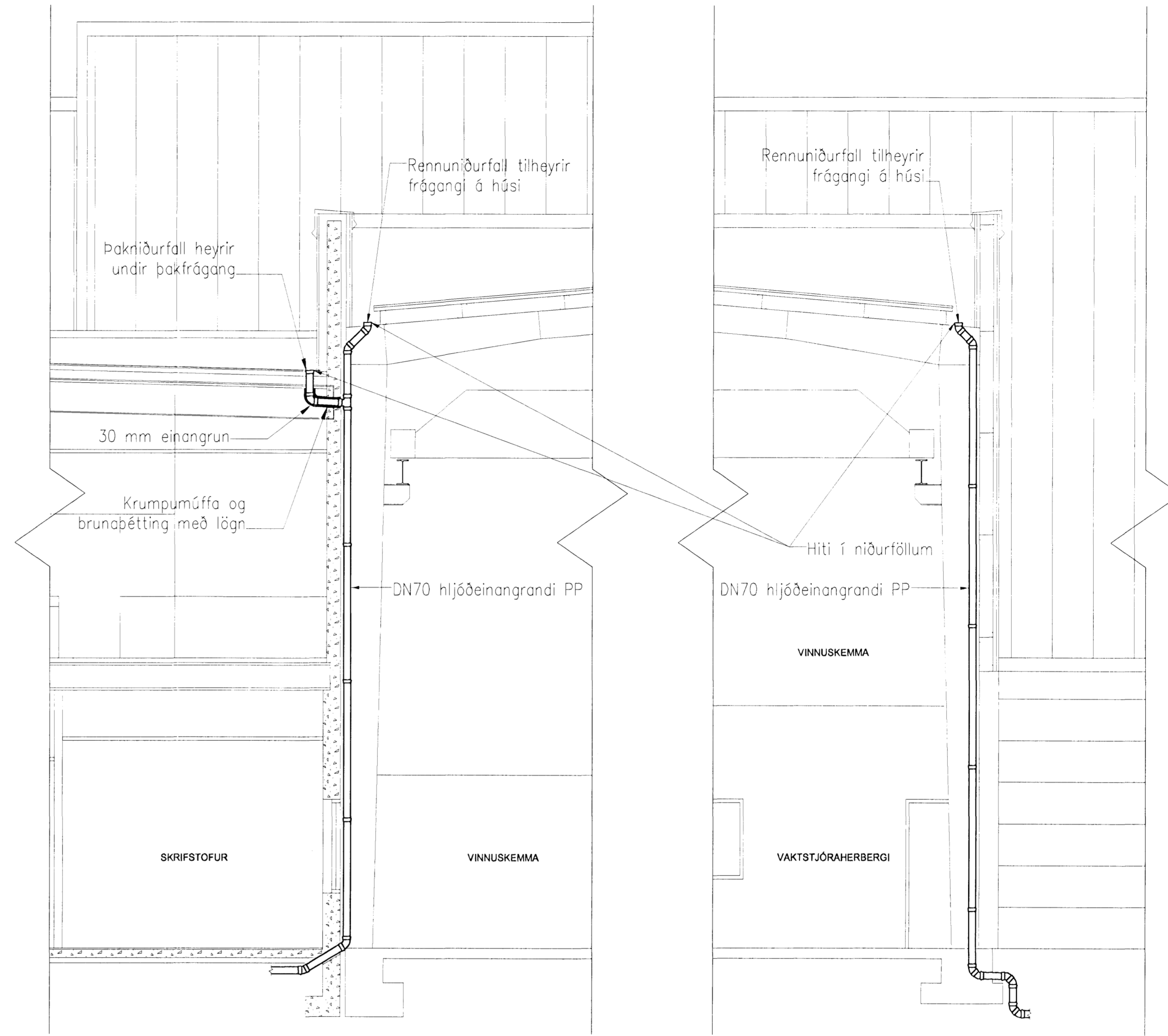
DÆMIGERÐUR FRÁGANÐUR ÞAKNIÐURFALLA Í VINNUSKEMMU, 1:50
