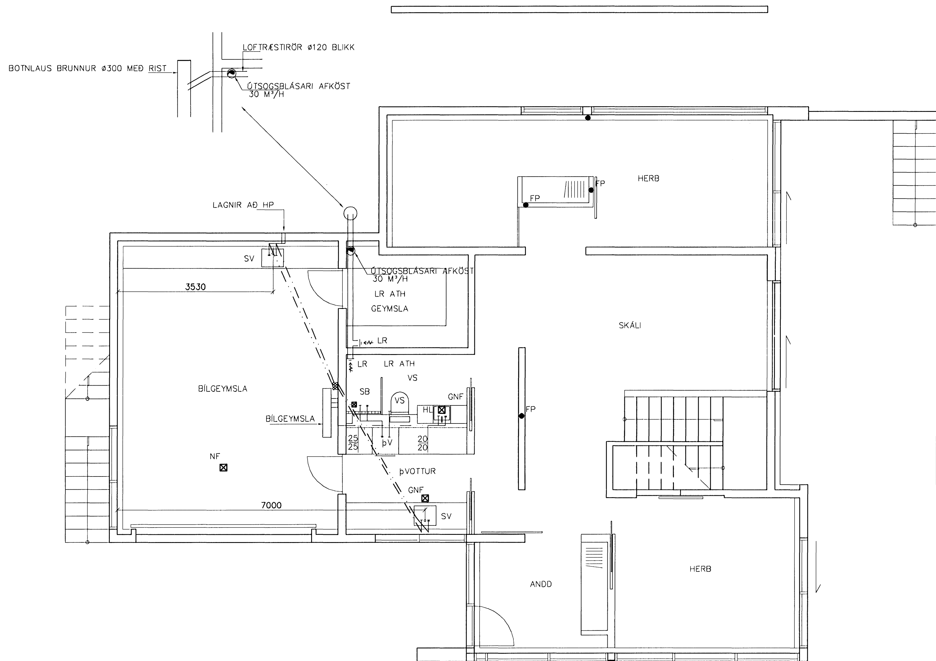
GRUNNMYND 1:50
