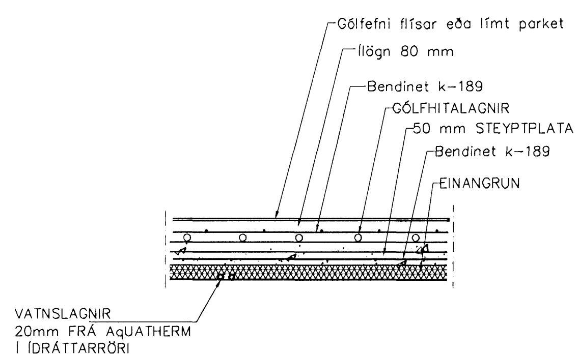
LAGNIR, SNIÐ, 1:20
