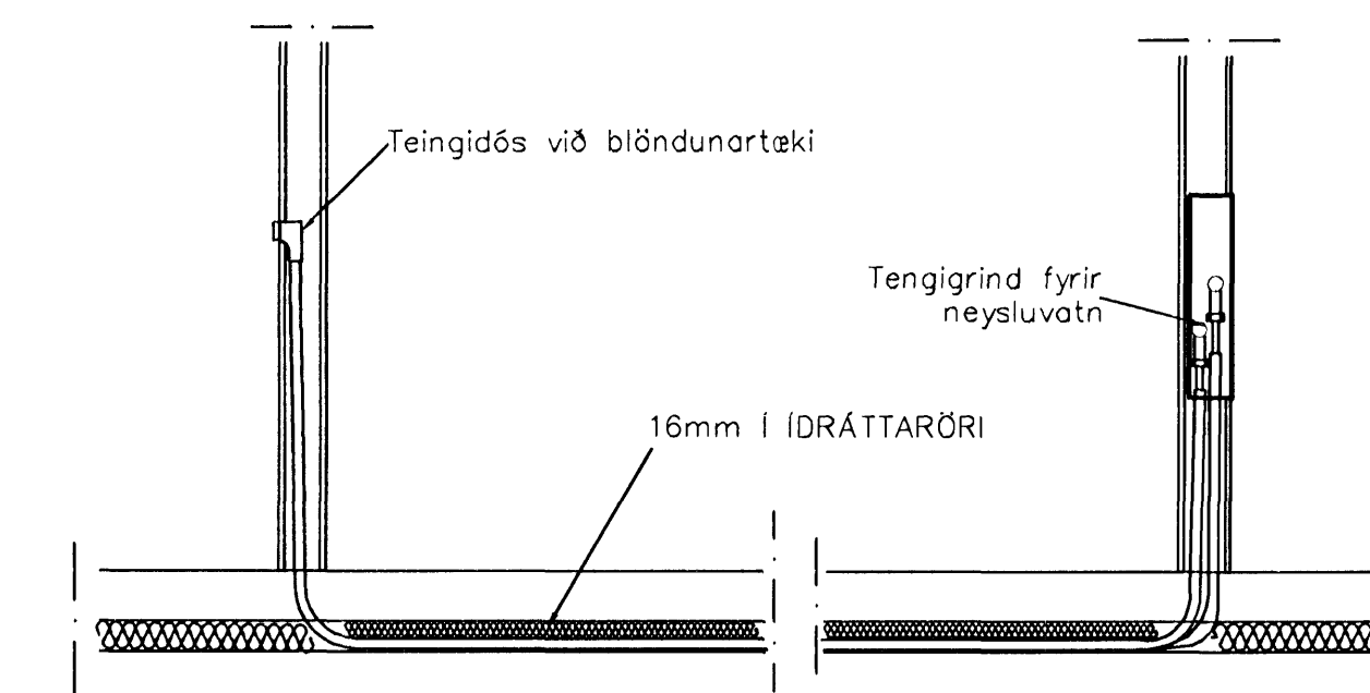
TENING NEYSLUVATNSLAGNA 1:20
