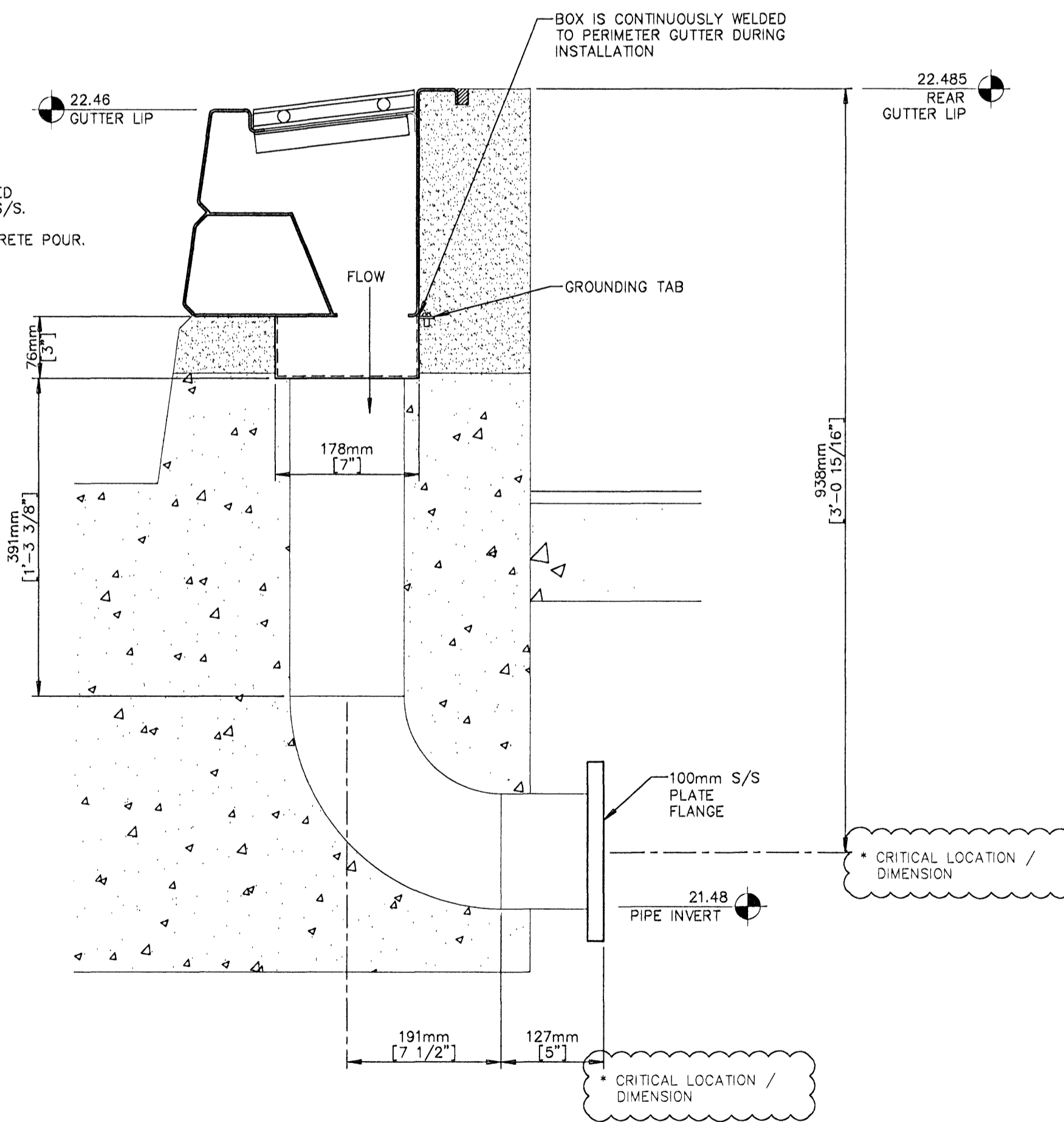
(D) 6.2 100mm GUTTER COLLECTOR BOX
