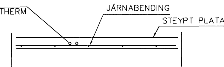
LAGNIR, SNIÐ, 1:20
