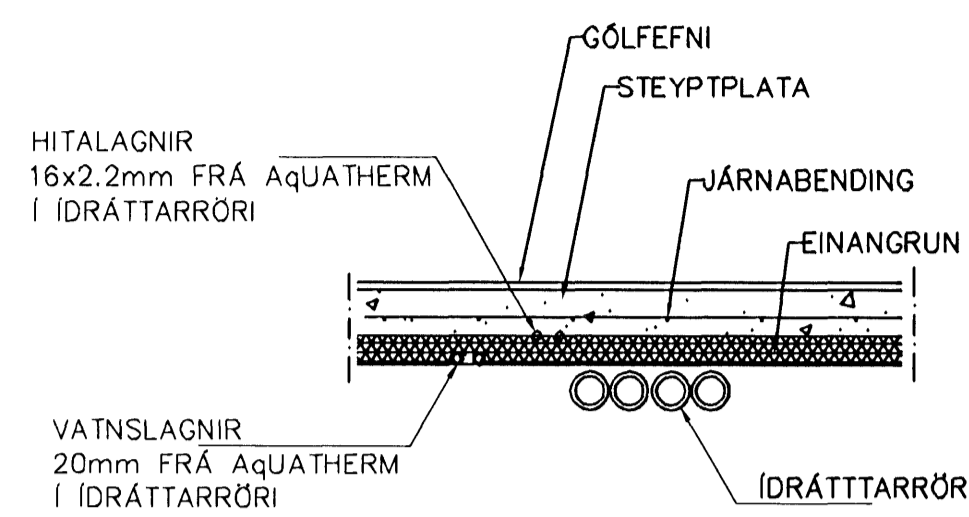
LAGNIR, SNIÐ, 1:20
