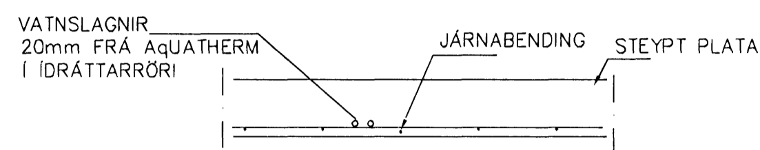
LAGNIR, SNIÐ, 1:20
