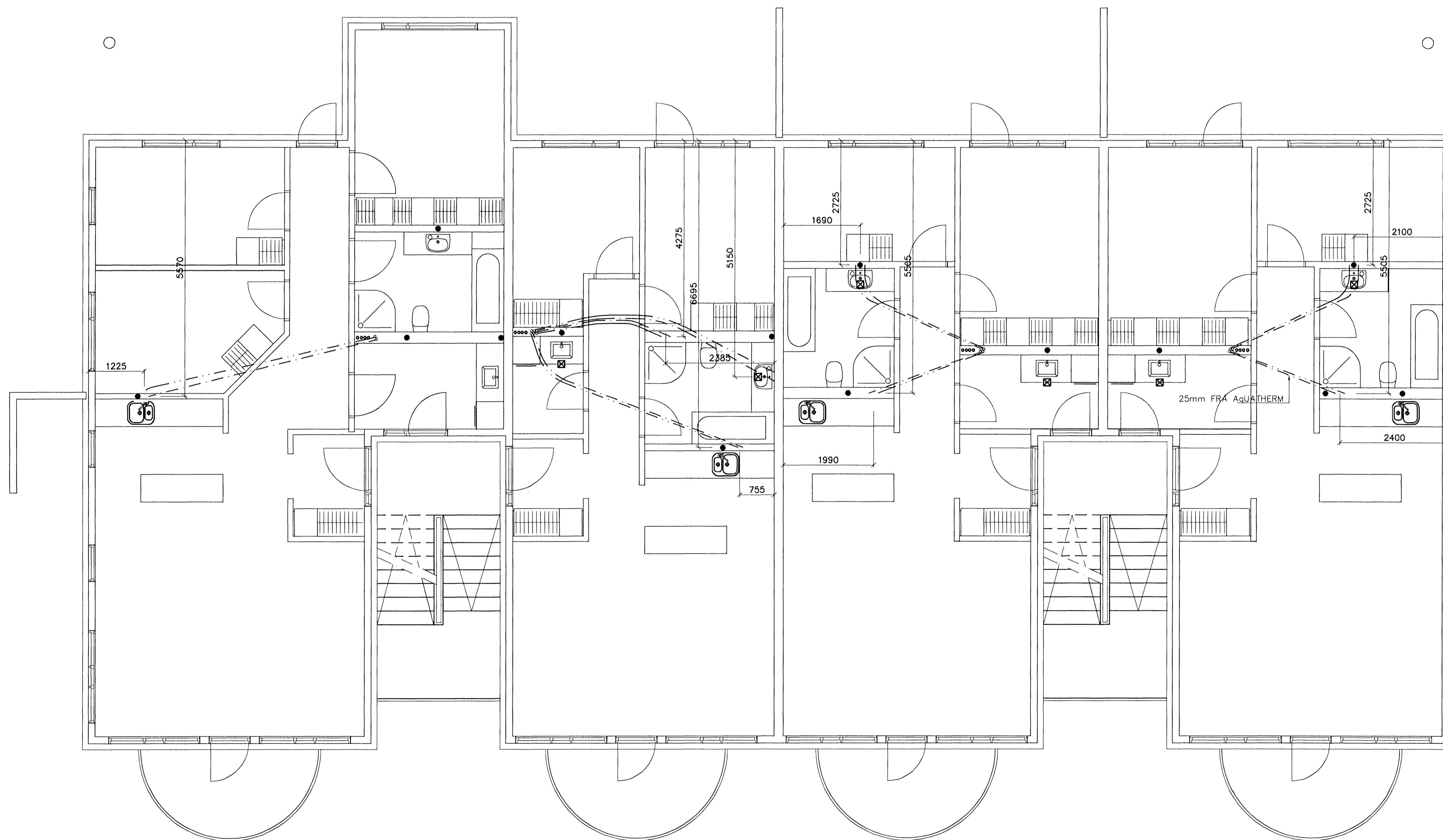
GRUNNMYND 3 HÆÐAR 1:50
