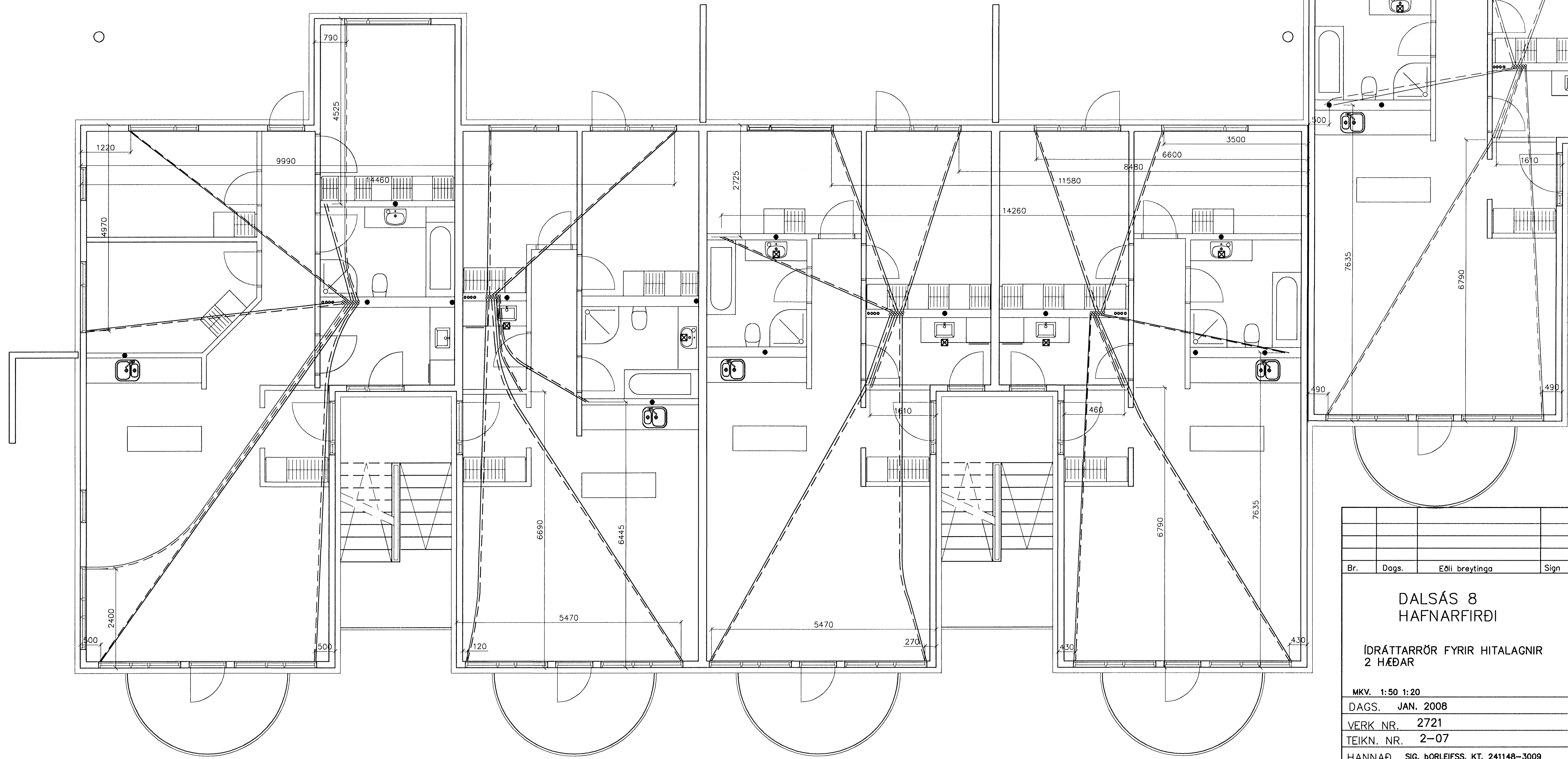
GRUNNMYND 2 HÆÐAR 1:50
