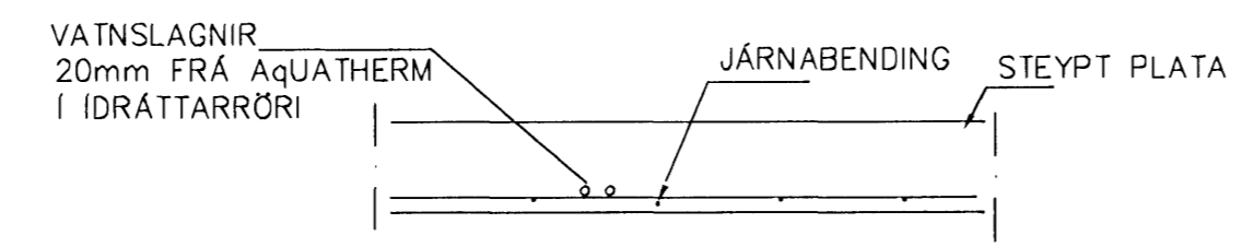
LAGNIR, SNIÐ, 1:20
