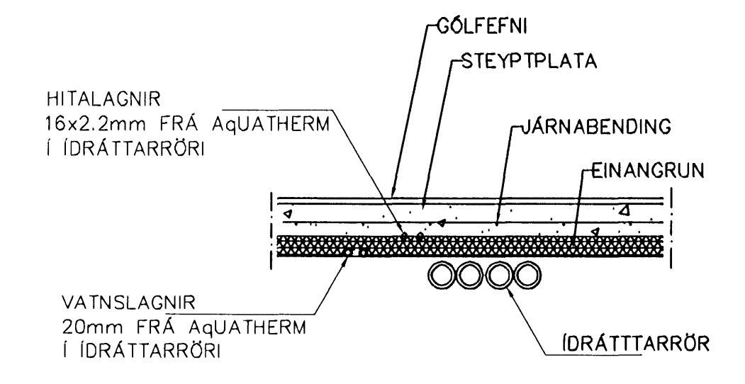
LAGNIR, SNIÐ, 1:20
