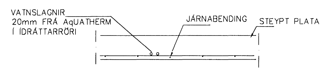
LAGNIR, SNIÐ, 1:20
