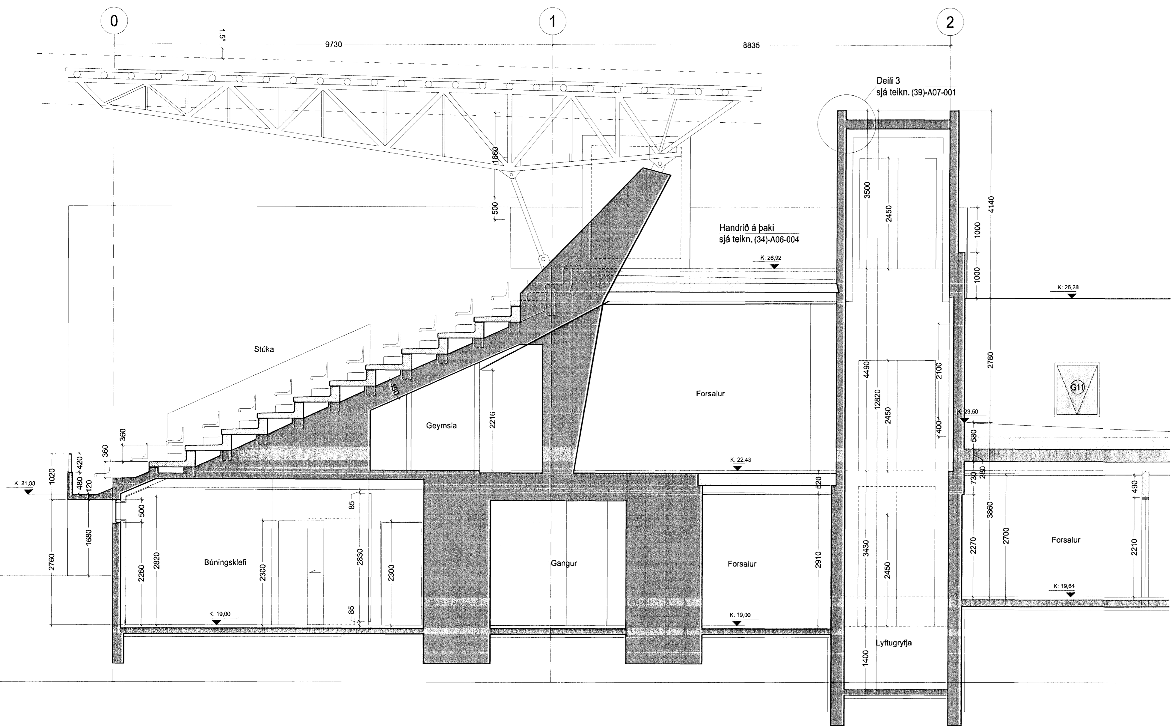
SNID E-E í mkv. 1:50
