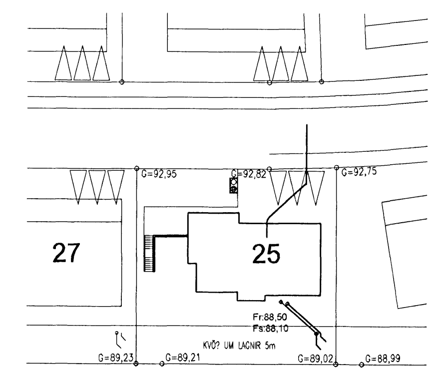
Afstöðumynd 1:500
