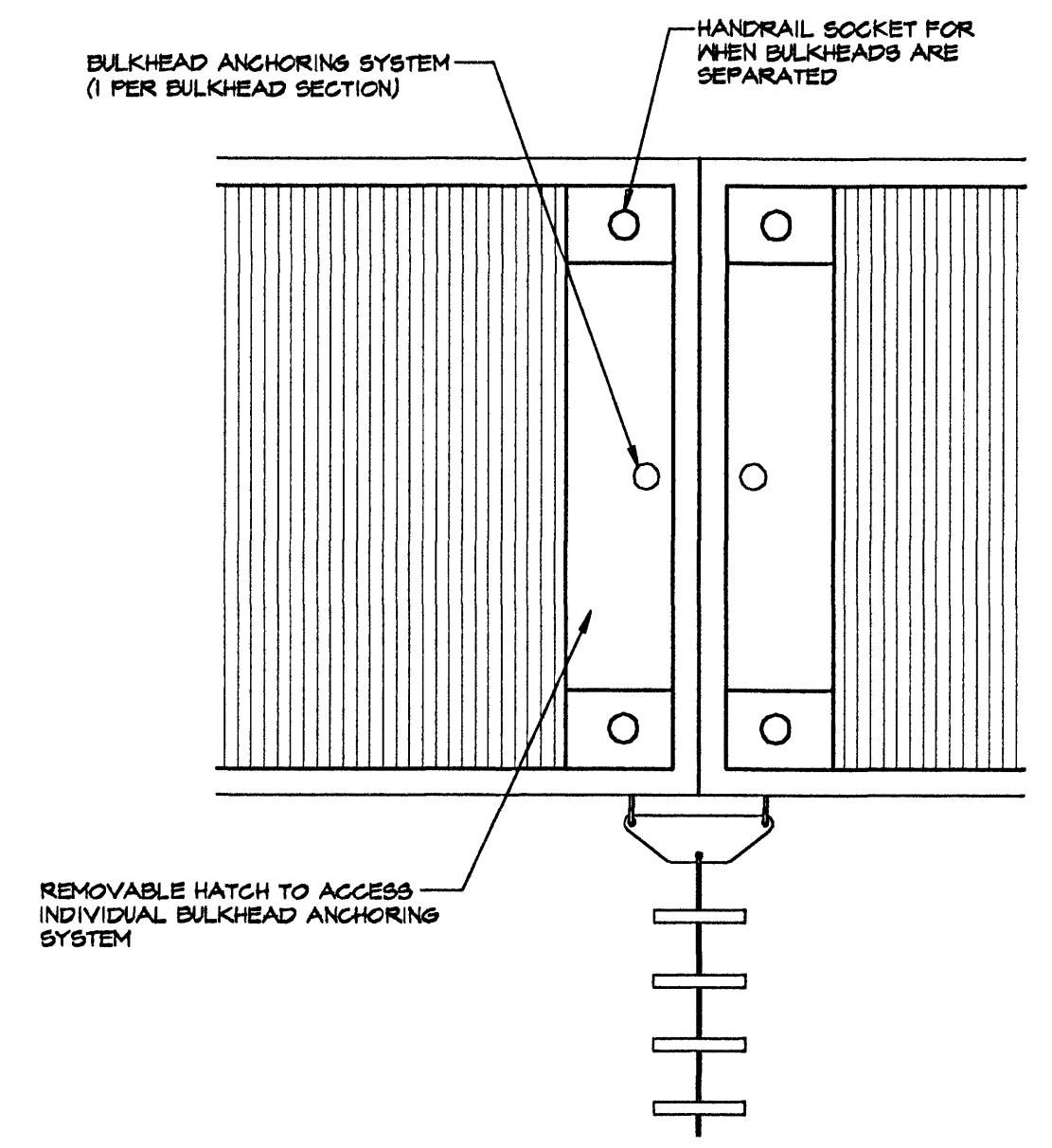
(D) PLAN VIEW REMOVABLE HATCH
