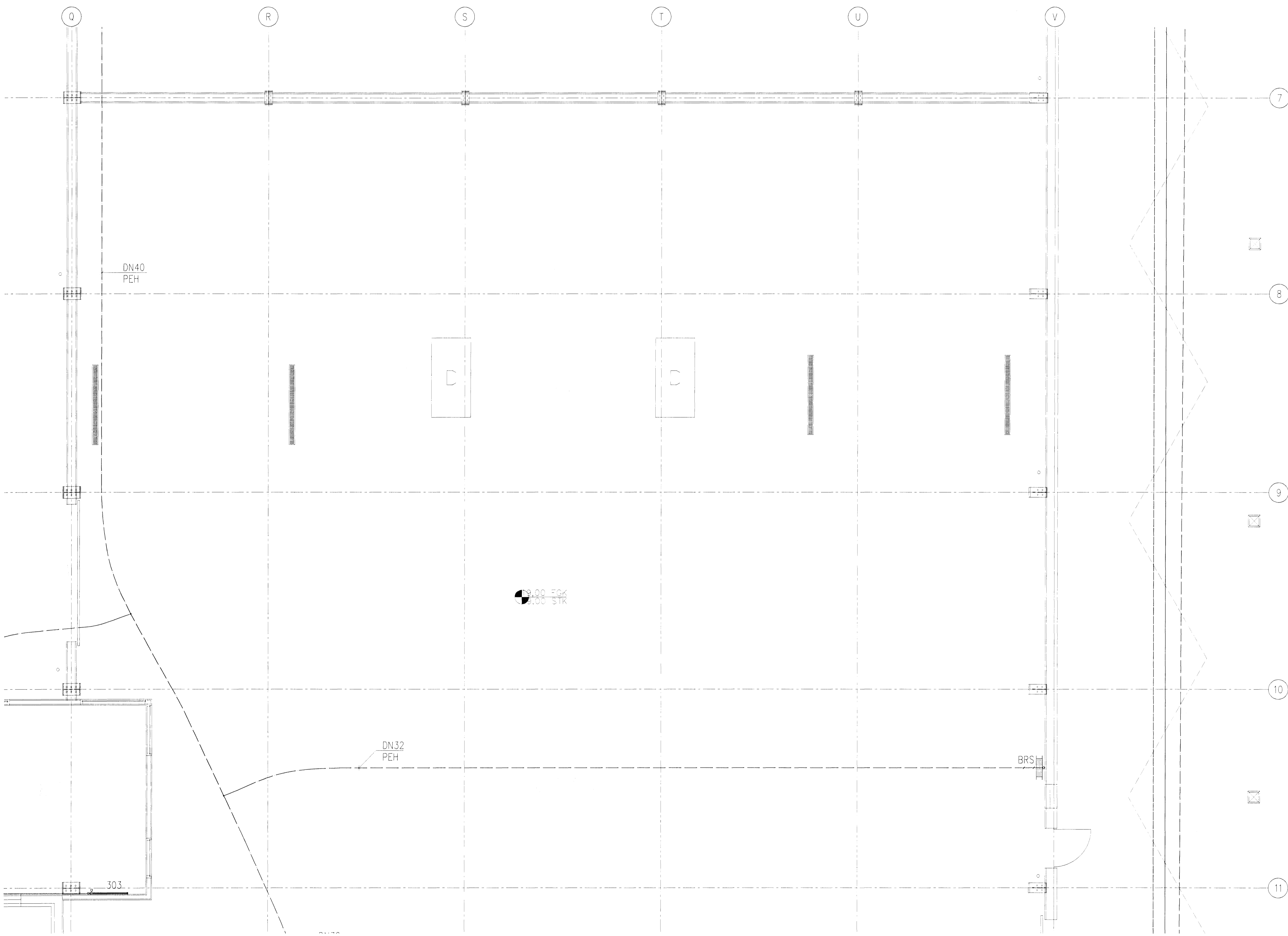
LAGNIR 1. HÆÐ 1:50
