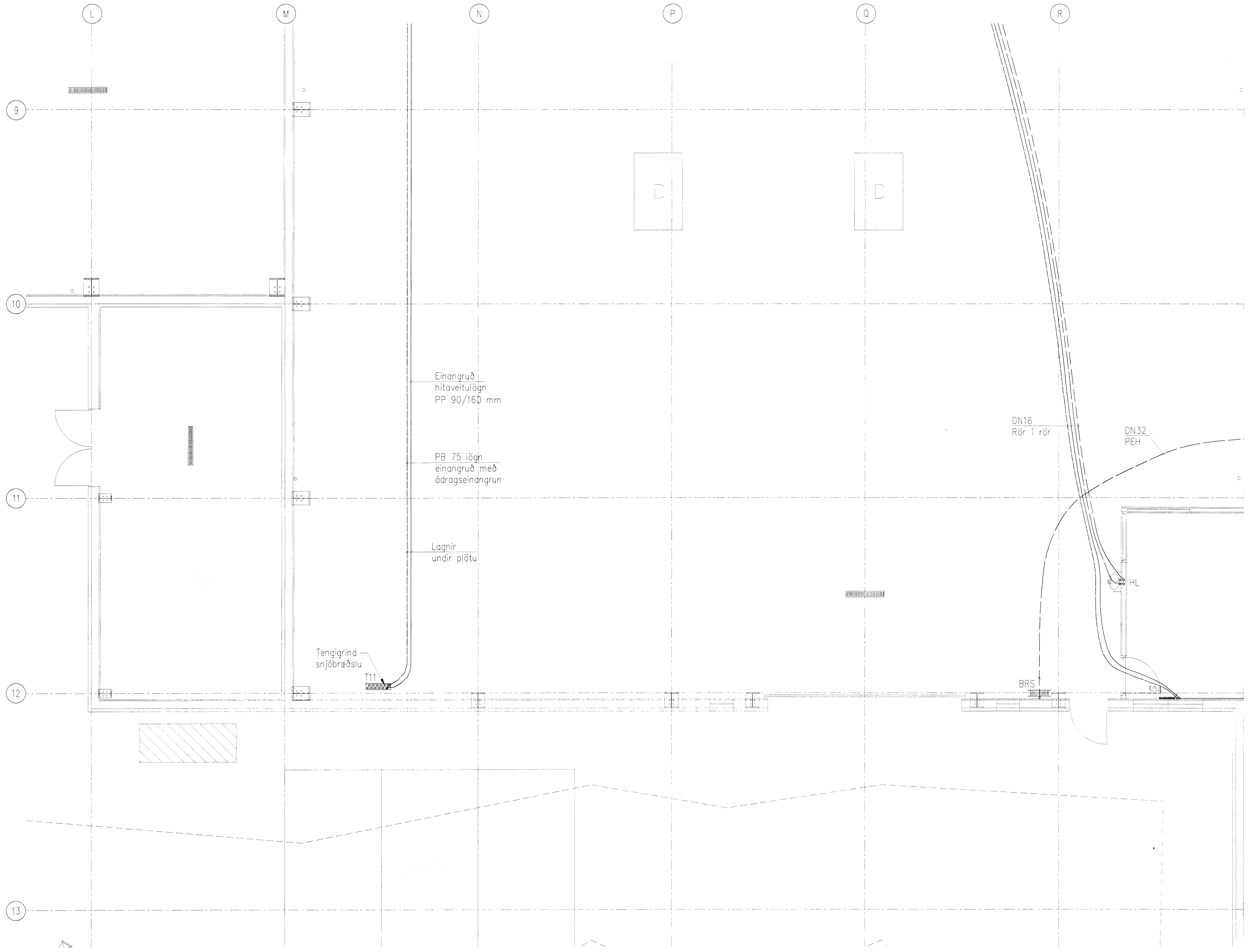
LAGNIR 1. HÆÐ 1:50
