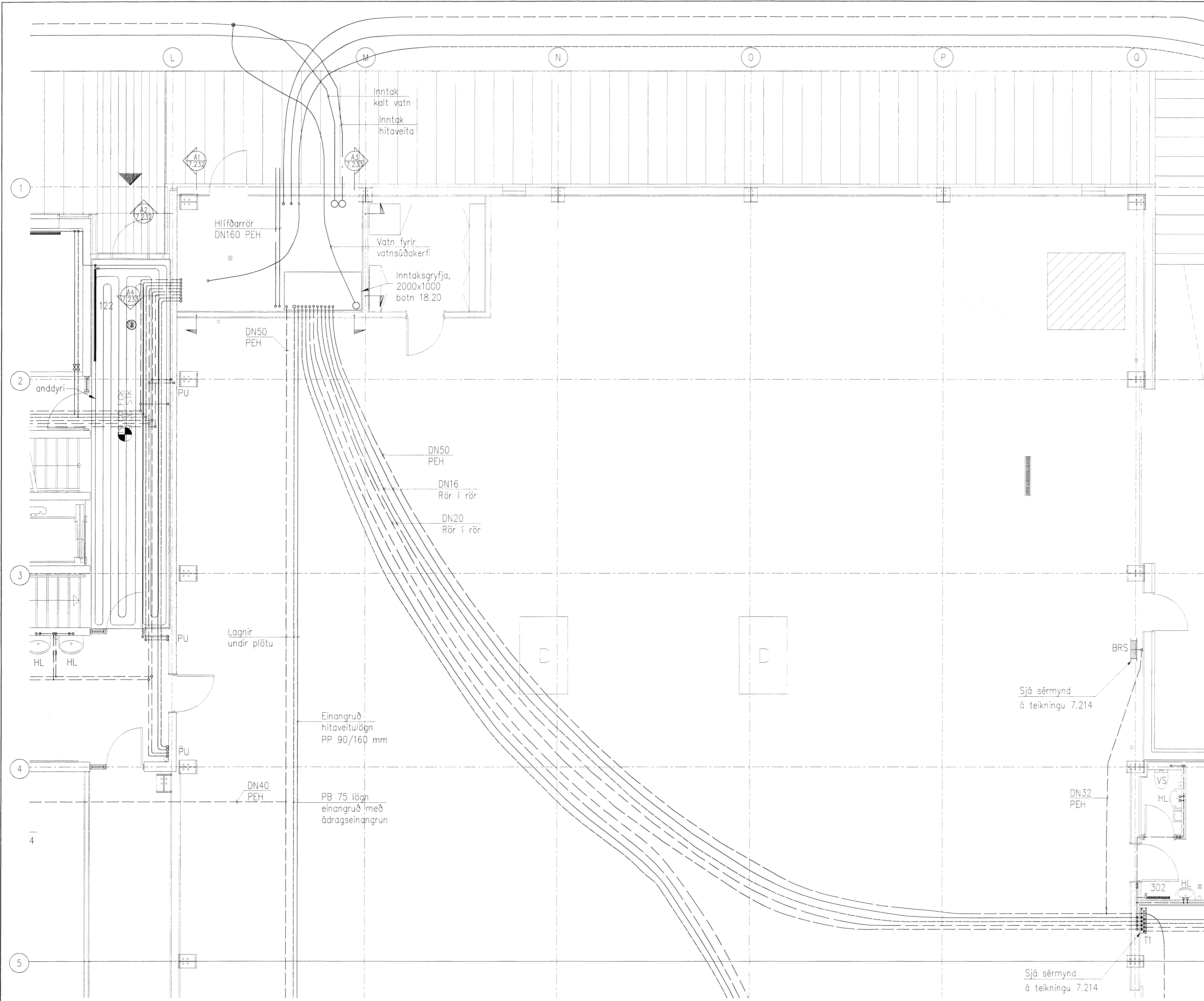
LAGNIR 1. HÆÐ 1:50
