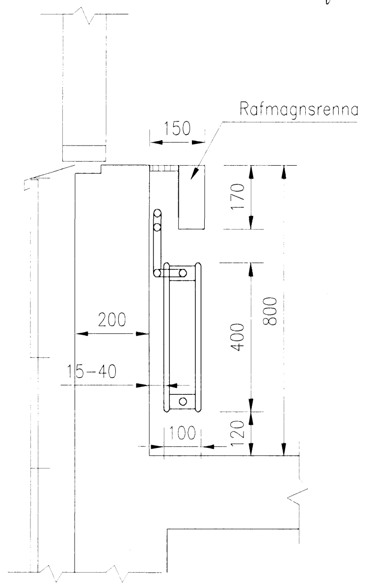
DÆMIGERÐUR FRÁGANGUR Á OFNUM Kvarði 1:10
