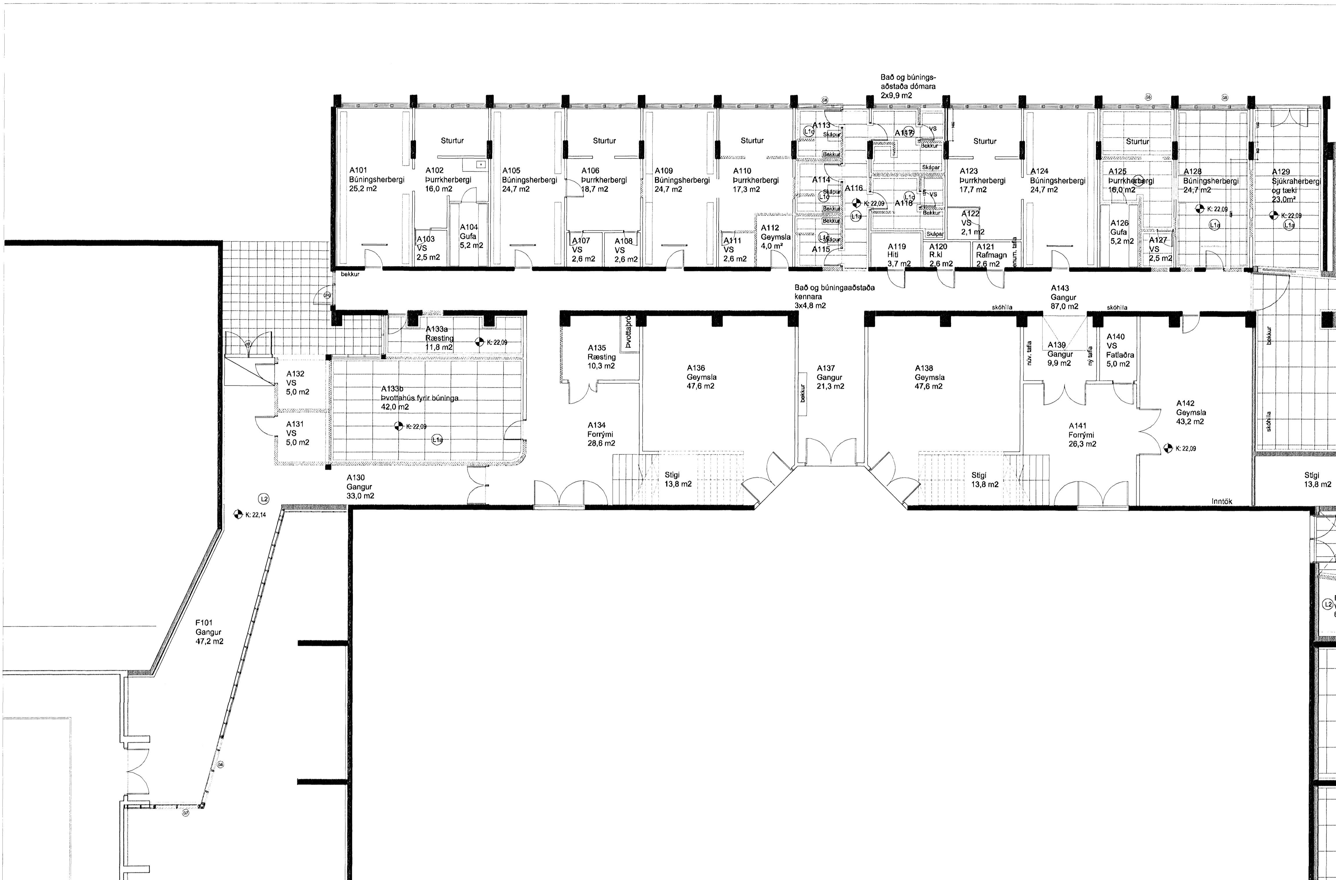
Grunnmynd 1.hæðar - loftaplan í mkv. 1:100
