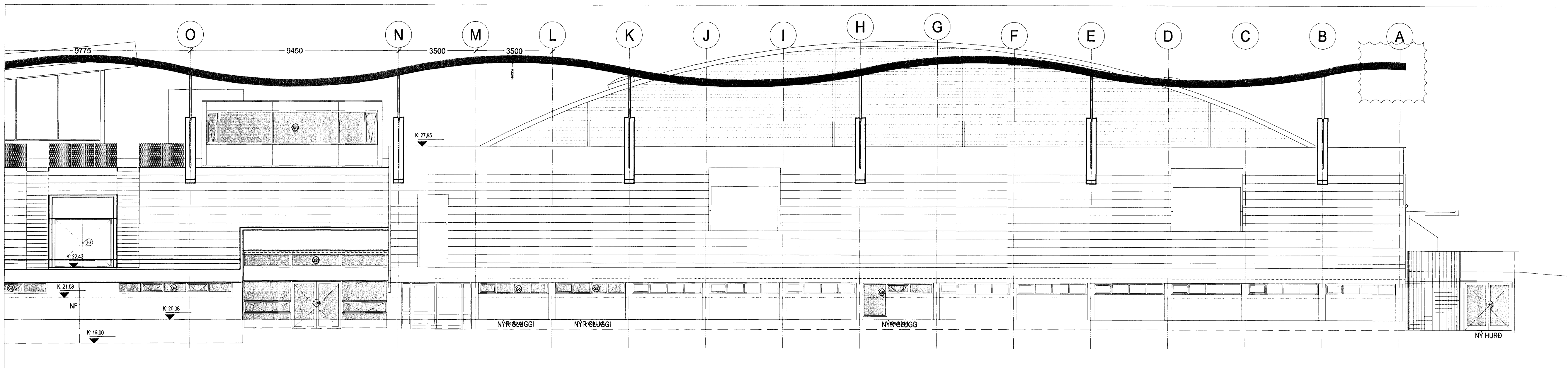
NORÐURHLIÐ A OG B HLUTA I mkv. 1:100
