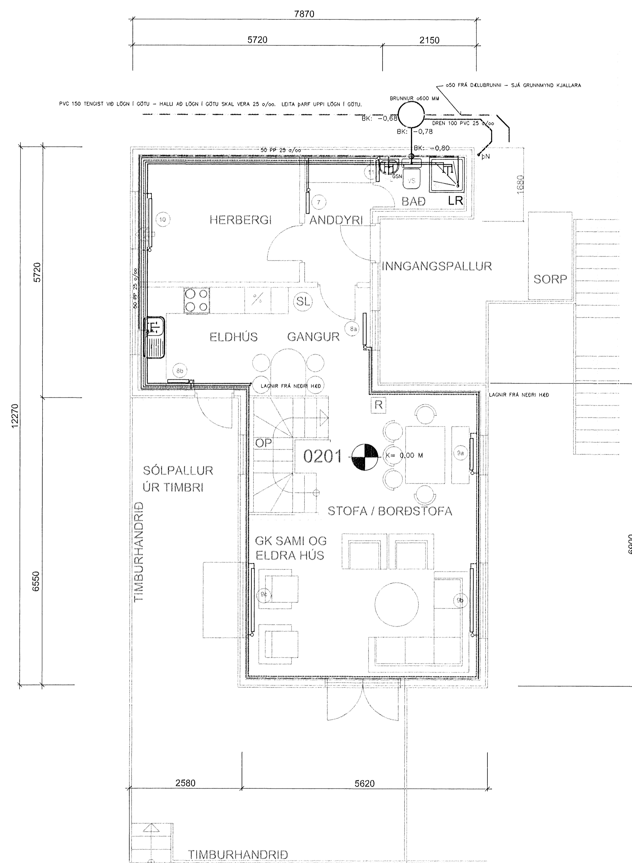
GRUNNMYND EFRÍ HÆÐAR
