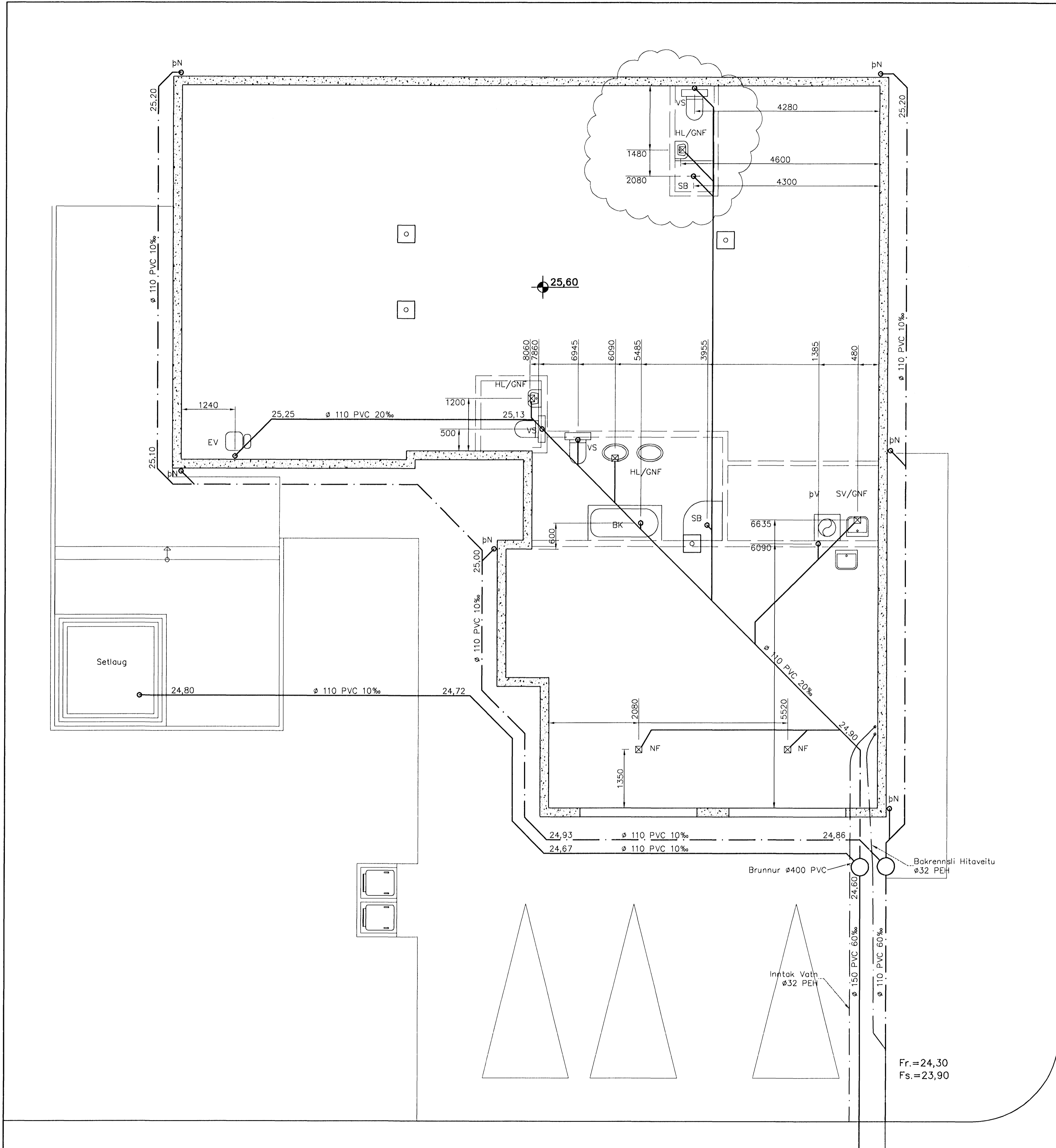
Grunnlagnir, Grunnmynd, 1:50
