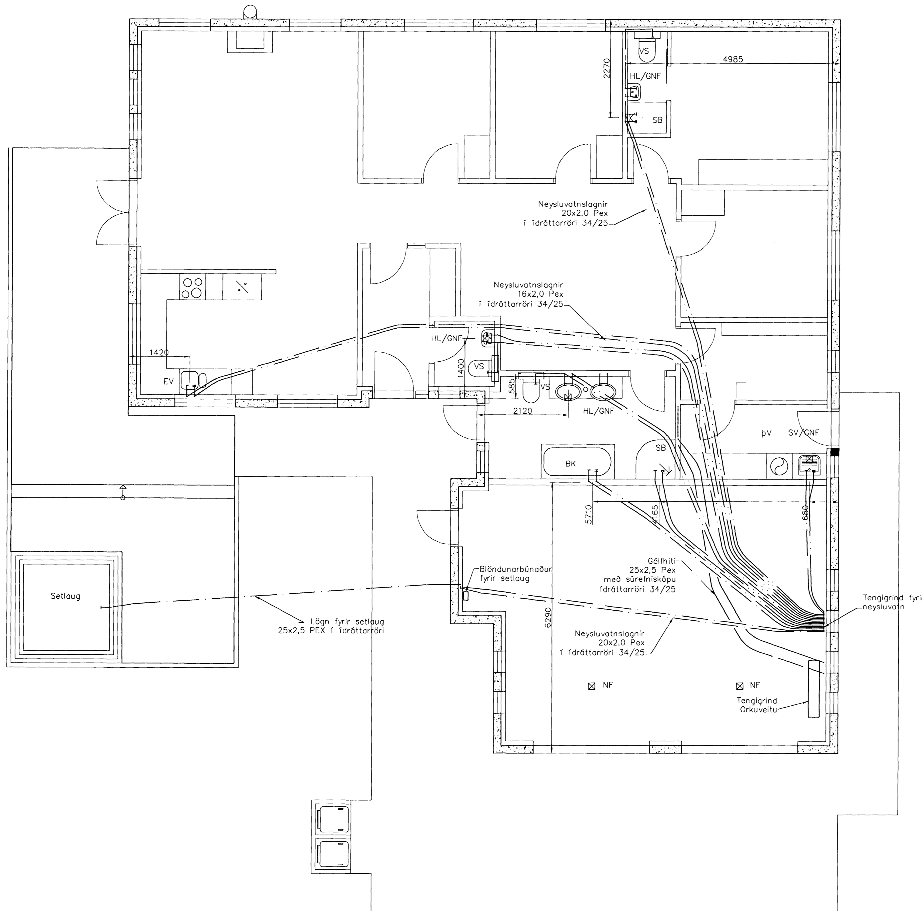
Neysluvatnslagnir, Grunnmynd, 1:50
