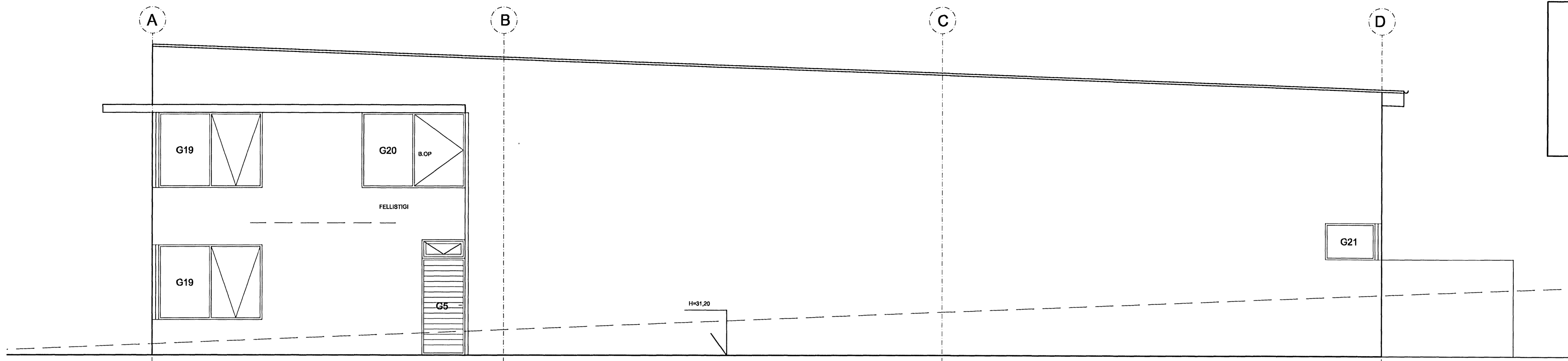
ÚTLIT Í NORÐUR M: 1/50
