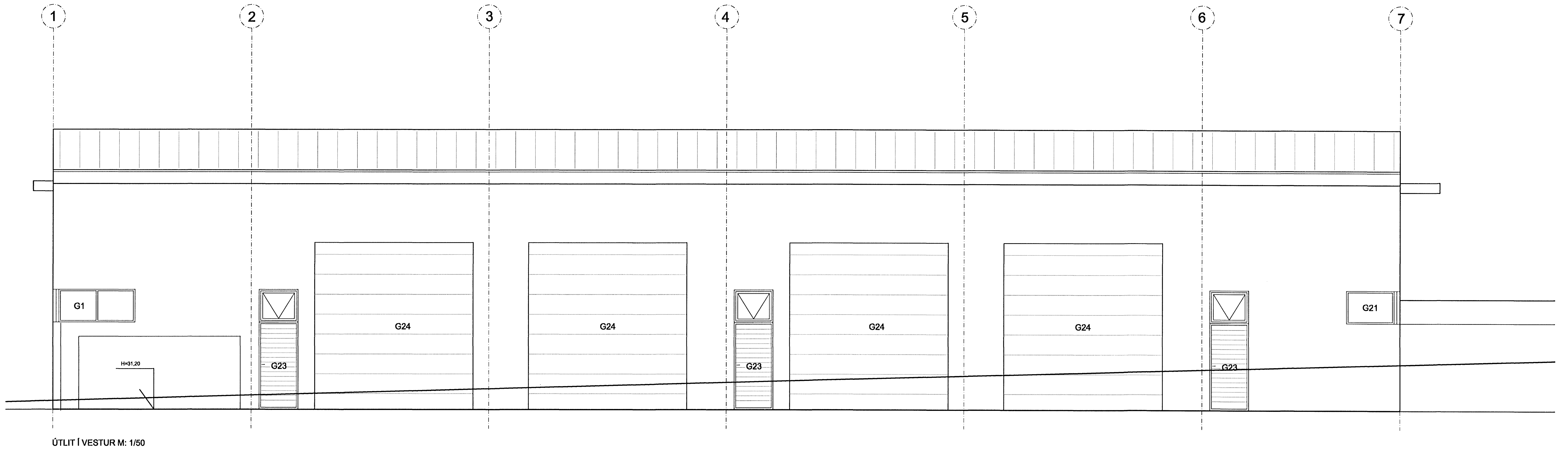
ÚTLIT Í VESTUR M: 1/50
