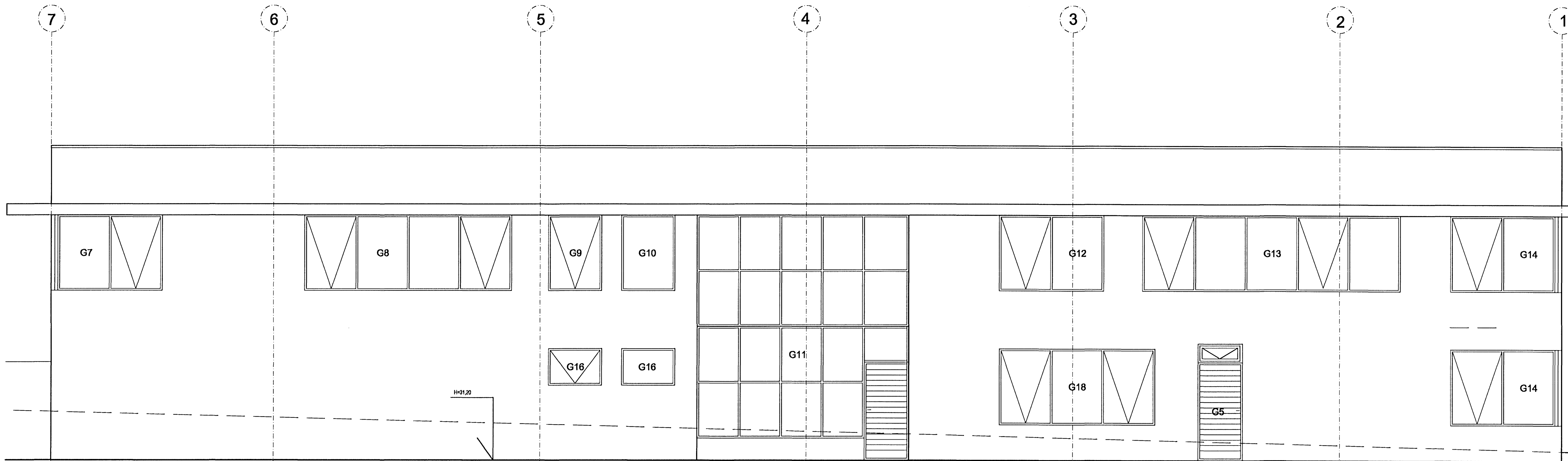
ÚTLIT Í AUSTUR M: 1/50
