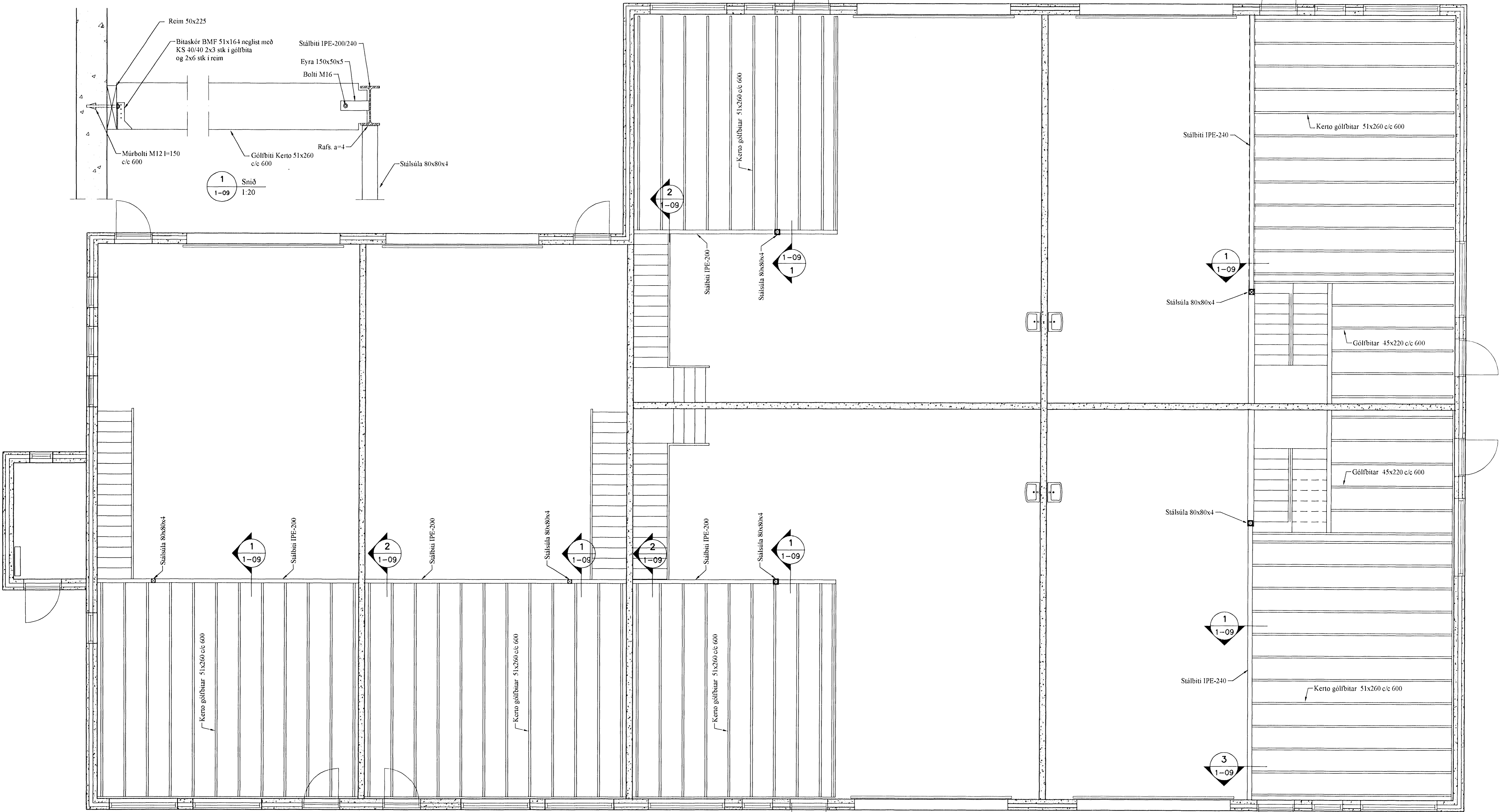
Grunnmynd, 1:50
