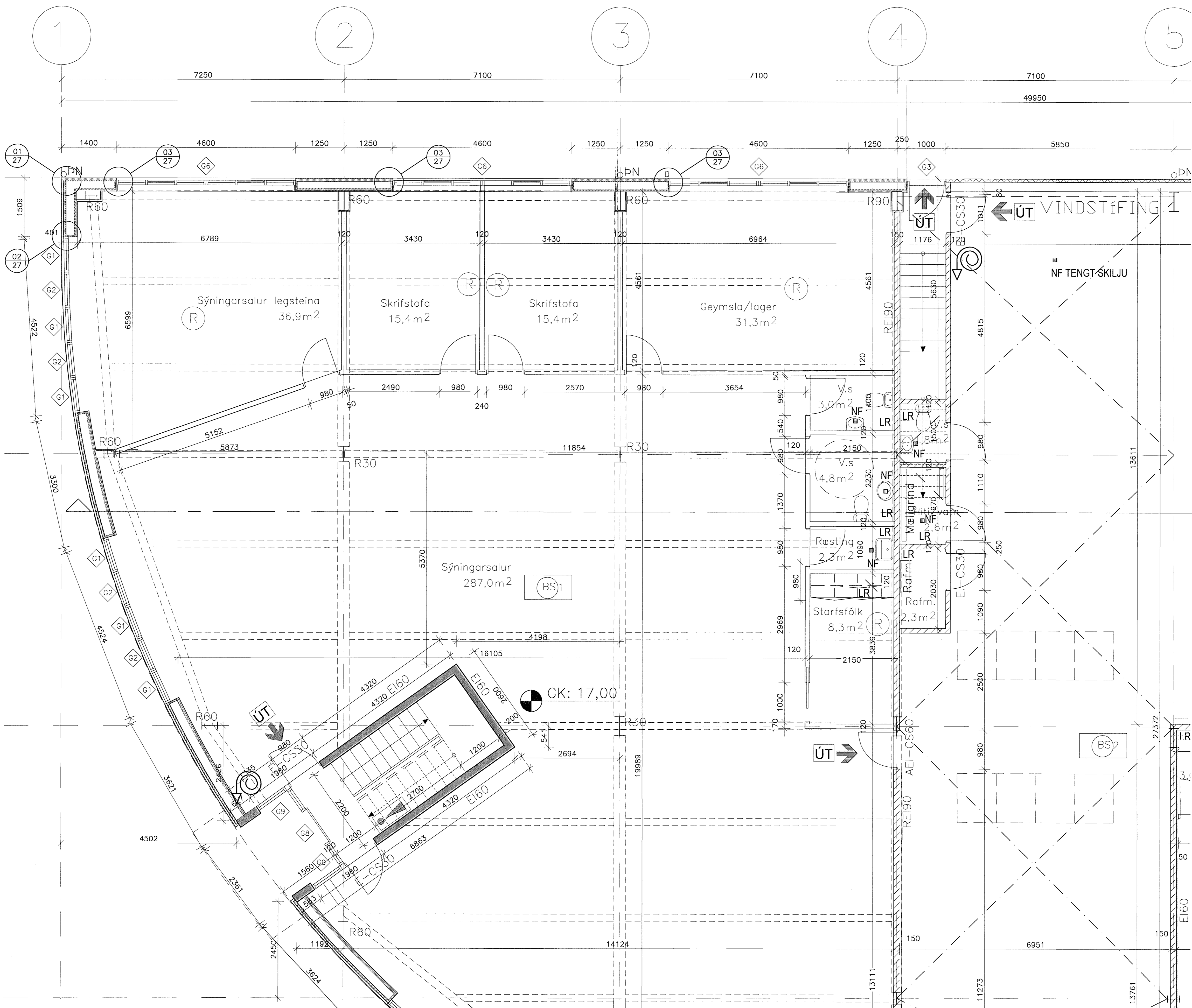
GRUNNMYND 1. HÆÐAR 1:50
