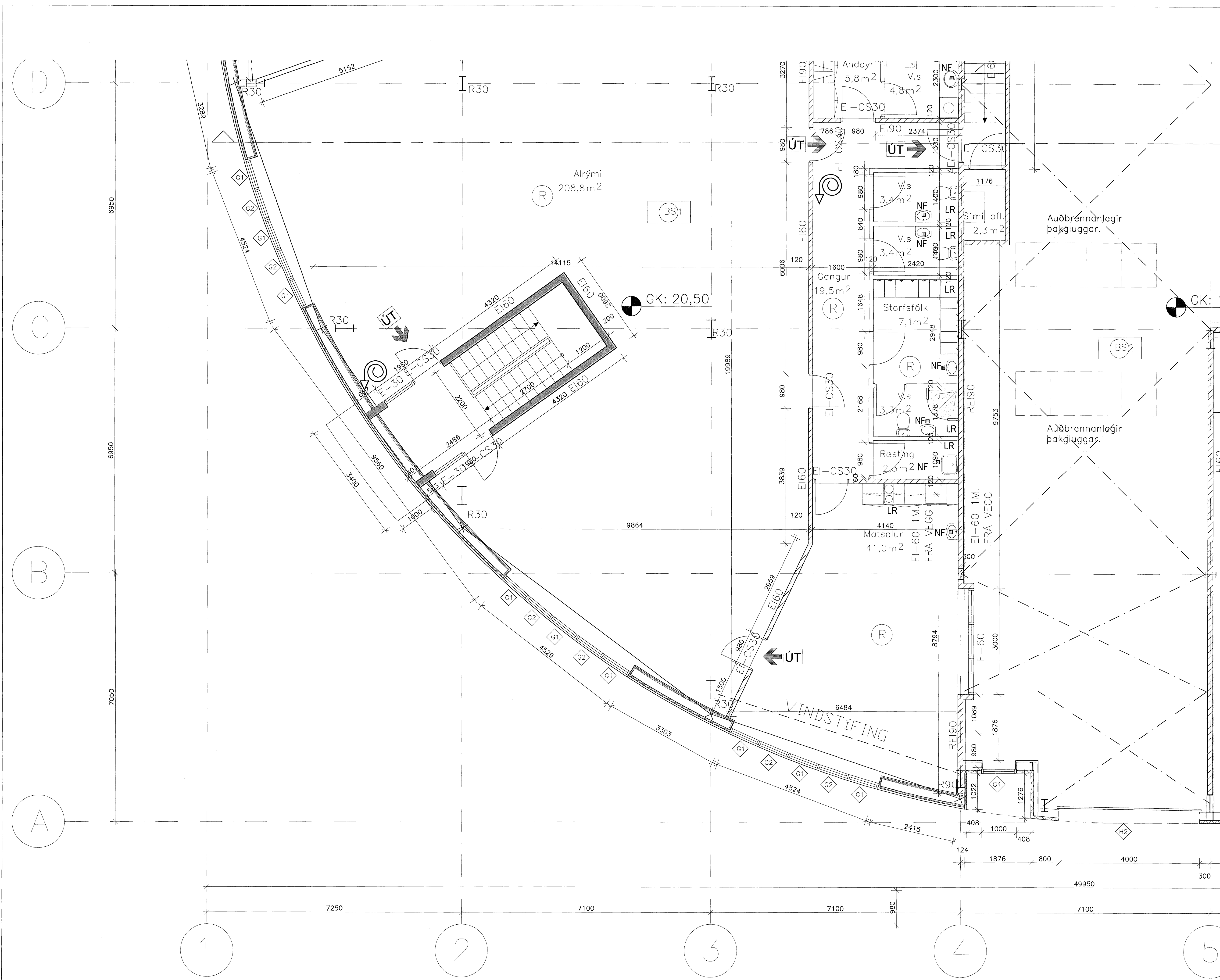
GRUNNMYND 2. HÆÐAR 1:50
