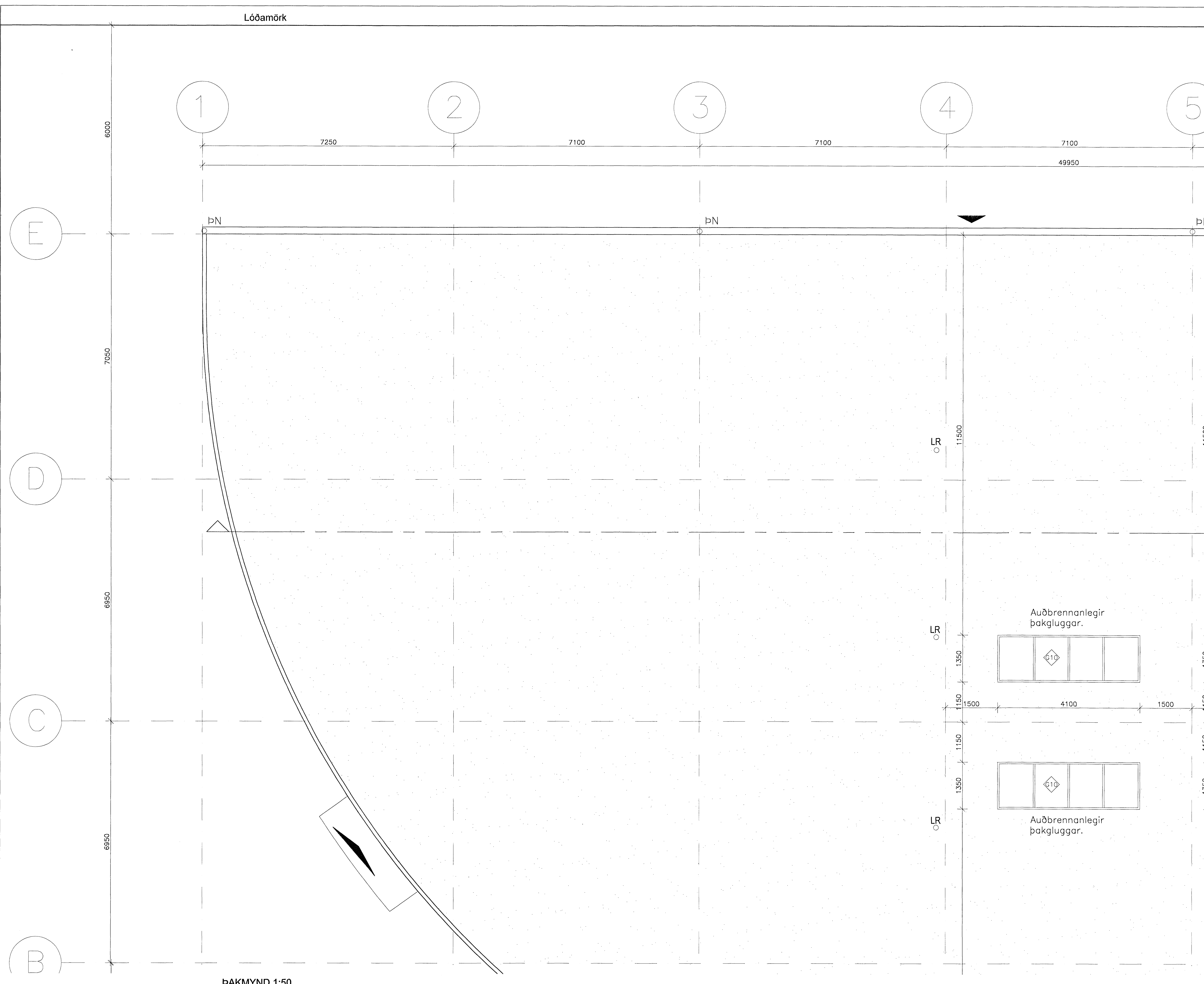
ÞAKMYND 1:50
