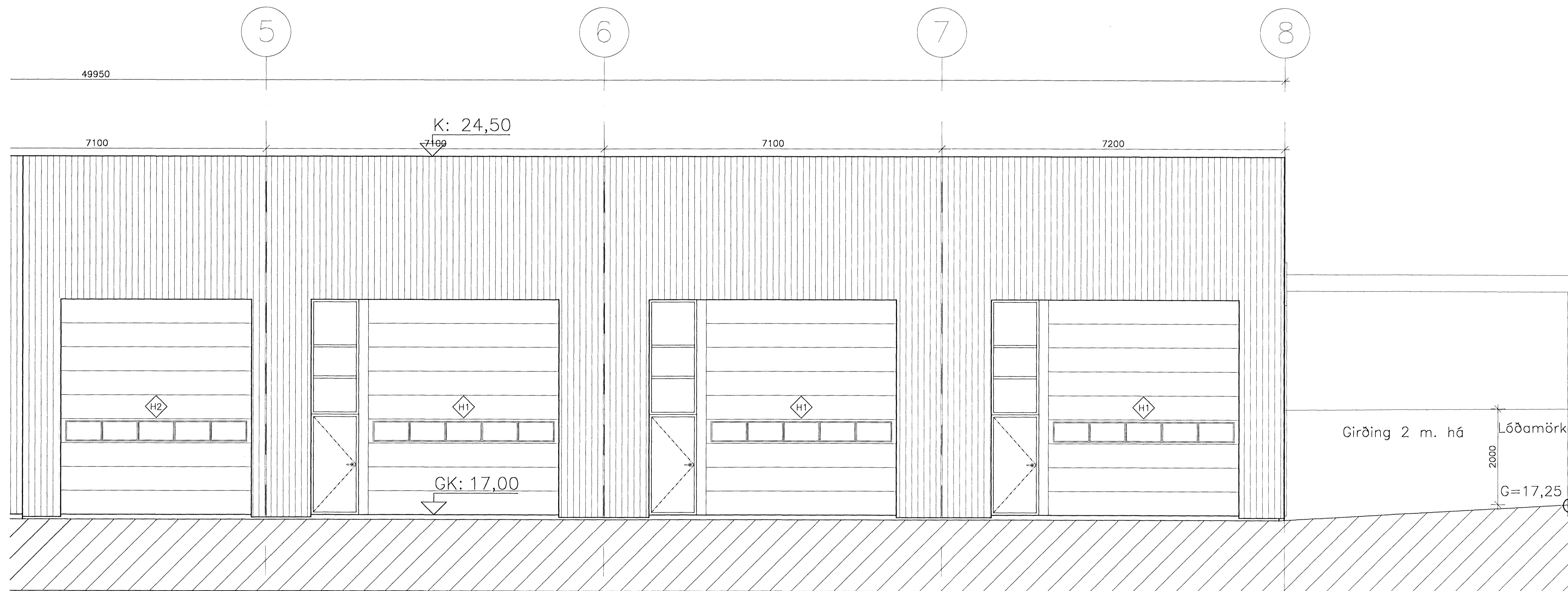
AUSTURHLIÐ 1:50
