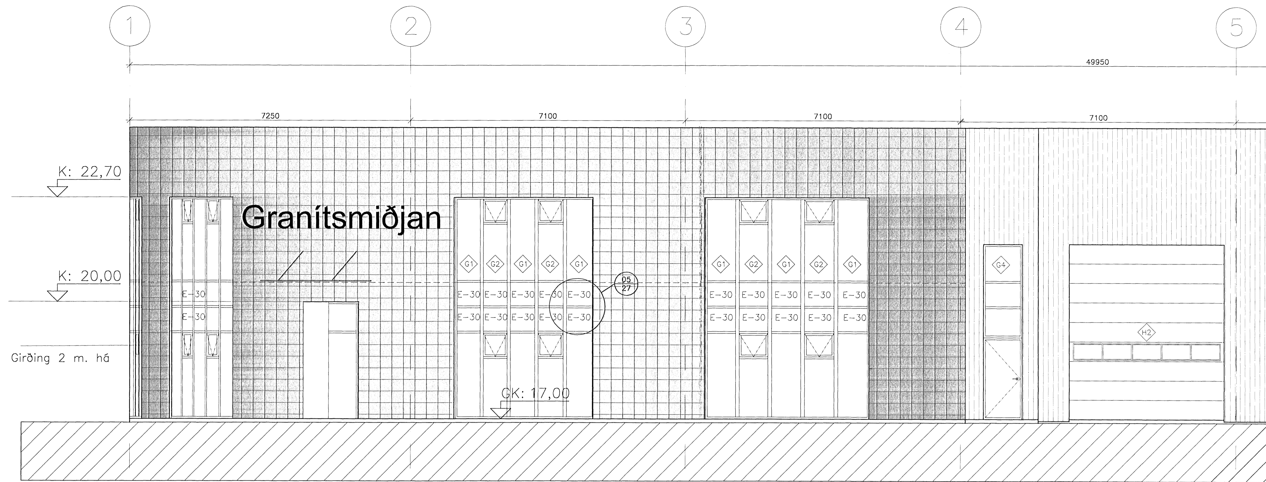
AUSTURHLIÐ 1:50
