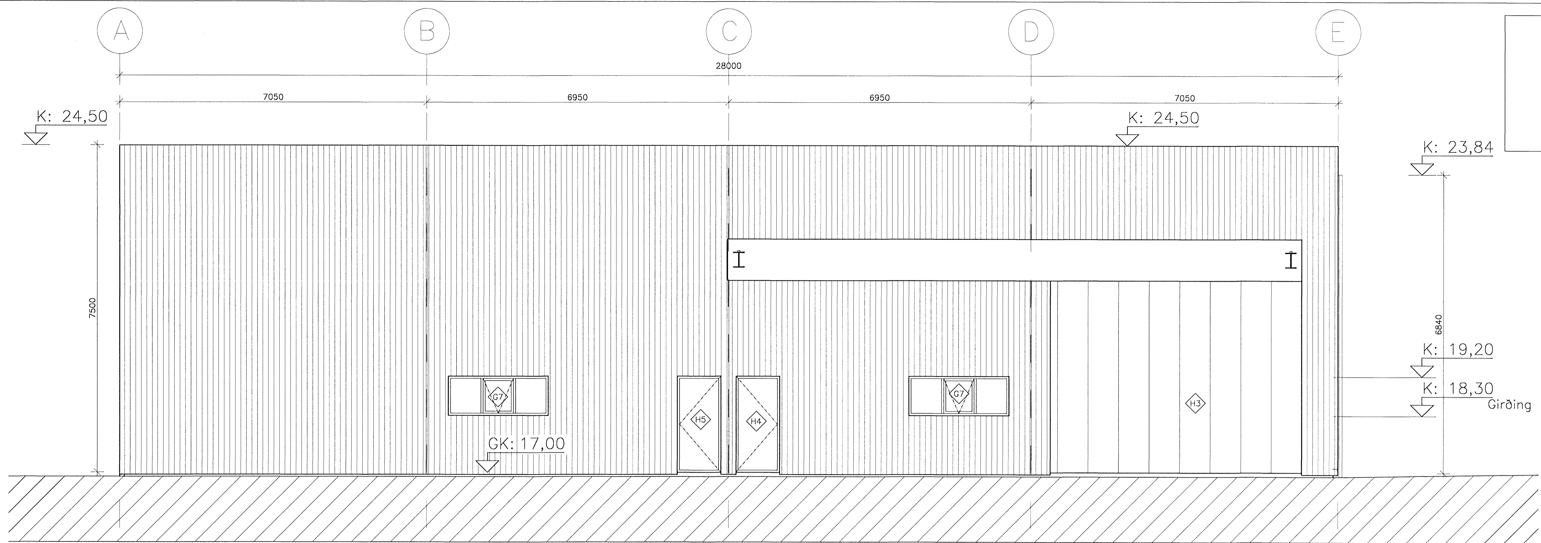
NORÐURHLIÐ 1:50
