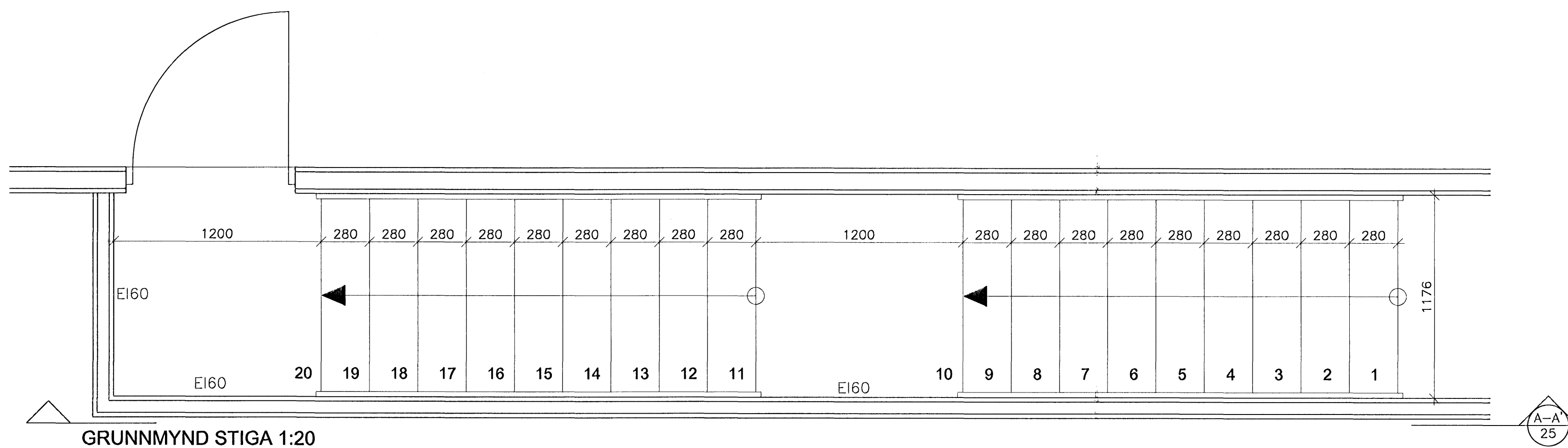
GRUNNMYND STIGA 1:20
