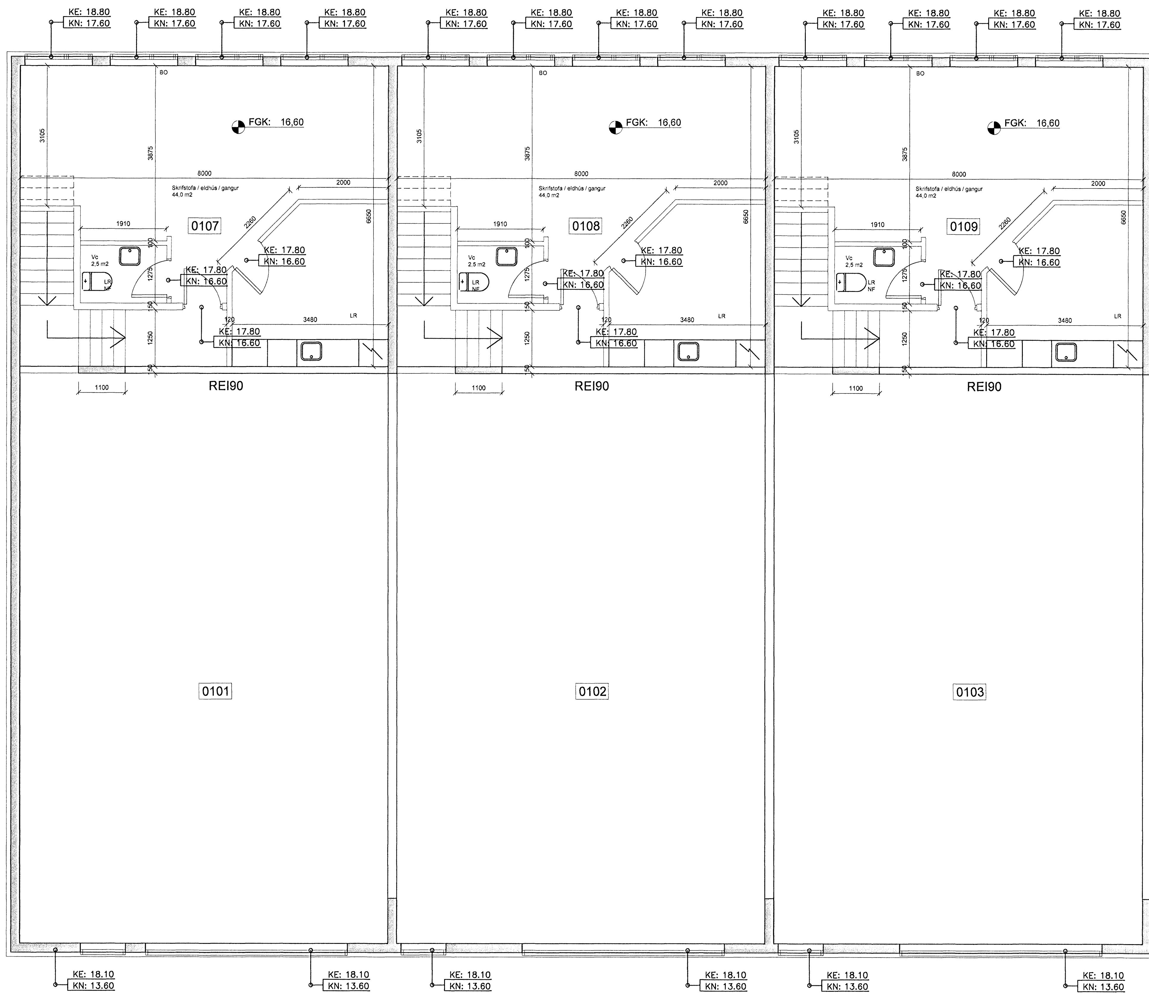
GRUNNMYND 2. HÆÐAR
