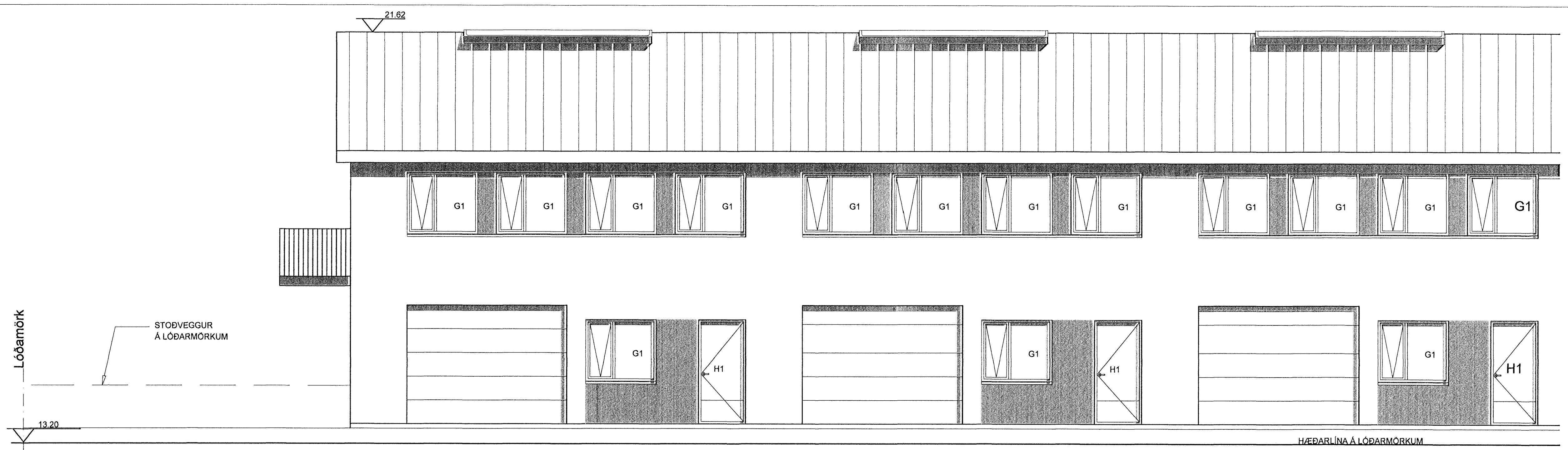
AUSTURHLIÐ, 1:50
