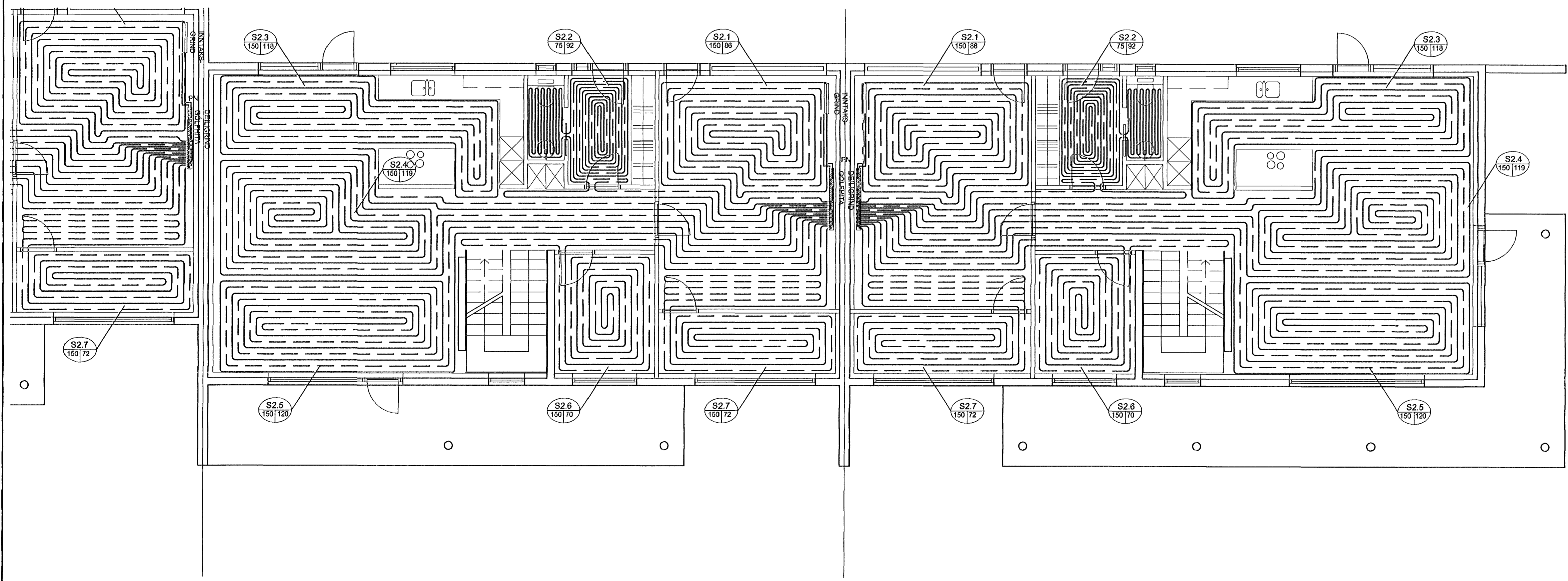
GRUNNMYND 2. HÆÐ, mkv. 1:50
