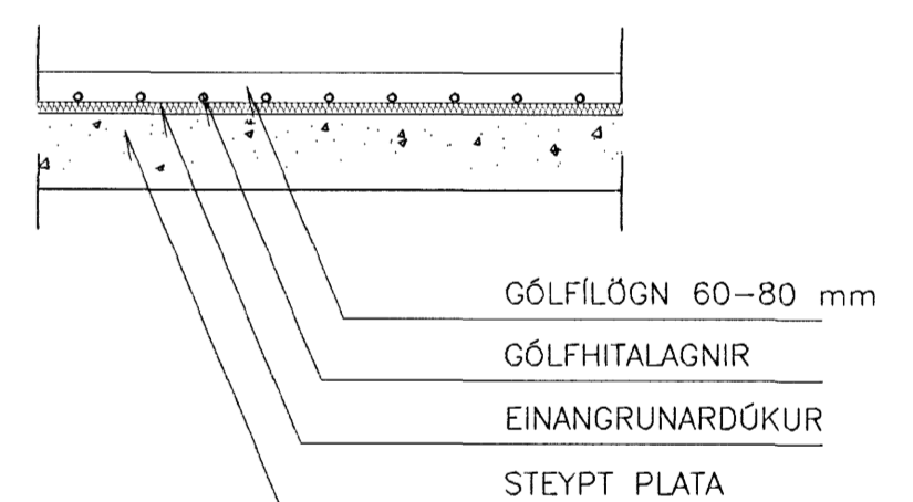
SNID Í MILLIPLÖTU Mkv. 1:20
