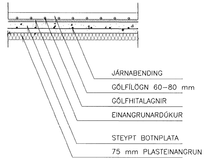
SNID Í BOTNPLÖTU Mkv. 1:20
