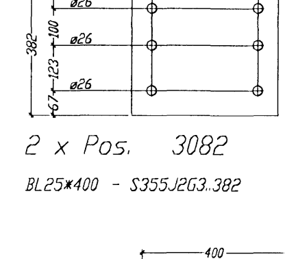
2 x Pos. 3082 BL25*400 - S355J2G3.382
