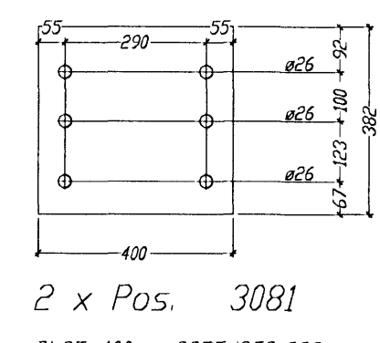
2 x Pos. 3081 BL25*400 - S355J2G3.382
