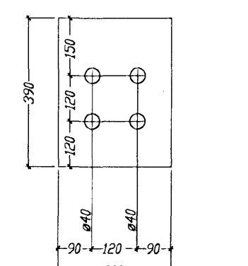
2 x Pos. 3091 BL35*390.300
