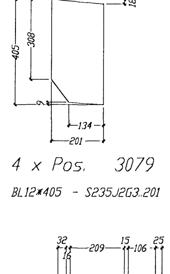
4 x Pos. 3079 BL12*405 - S235J2G3.201
