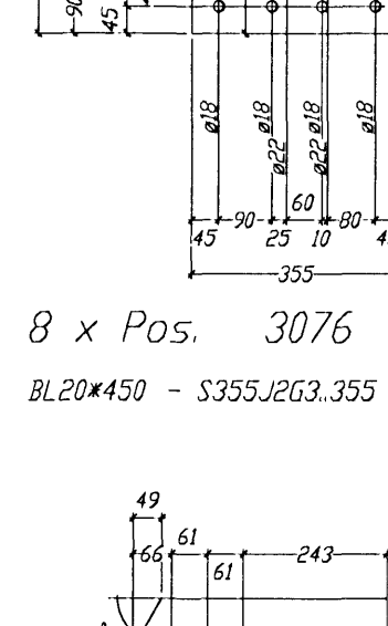
8 x Pos. 3076 BL20*450 - S355J2G3.355
