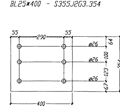
1 x Pos. 3084 BL25*400 - S355J2G3.354
