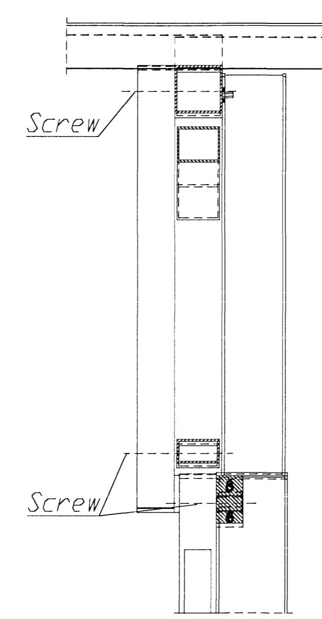
SECTION A-A Sc. 1:10
