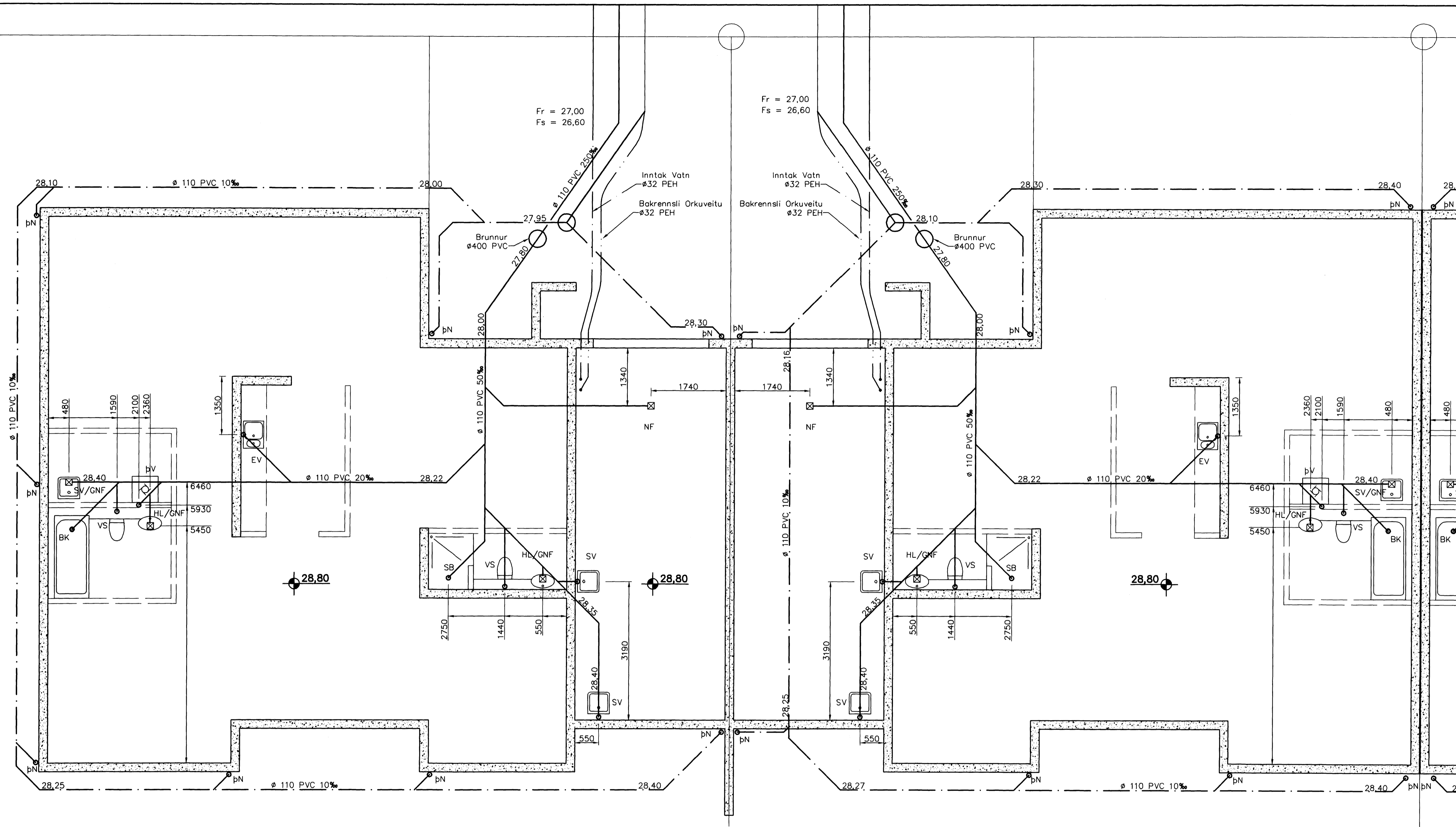
Grunnlagnir 1:50
